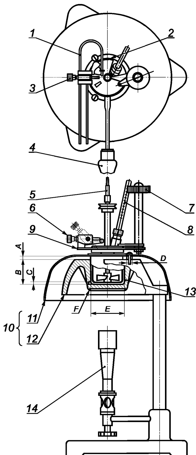
Рисунок А1.1 — Аппарат Пенски-Мартенса с закрытым тиглем
