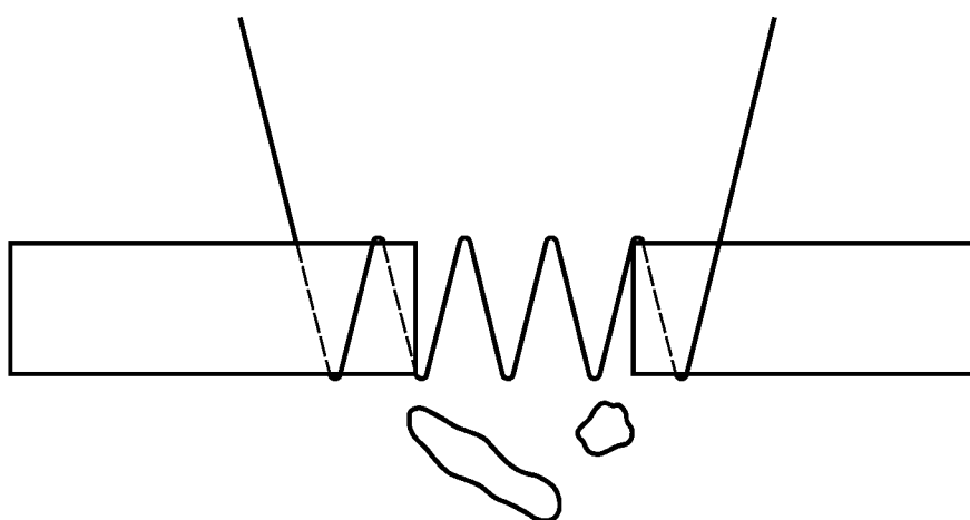
Рисунок С.3 — Частичное сквозное проплавление без воспламенения. Результат испытания — воспламенения нет
