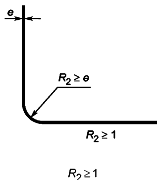
Рисунок А.2.1 — Зона распыления. Две перпендикулярные поверхности
