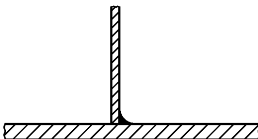
Рисунок А.2.3 — Зона распыления. Две перпендикулярные поверхности, соединенные сваркой
