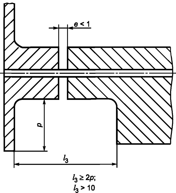
Рисунок А.12 — Шарнирное соединение
