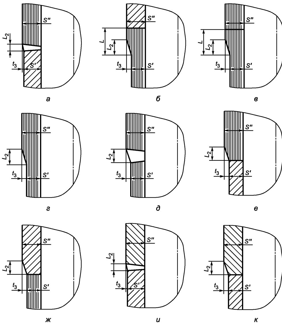
Рисунок 5.1 — Соединение цилиндрических обечаек
