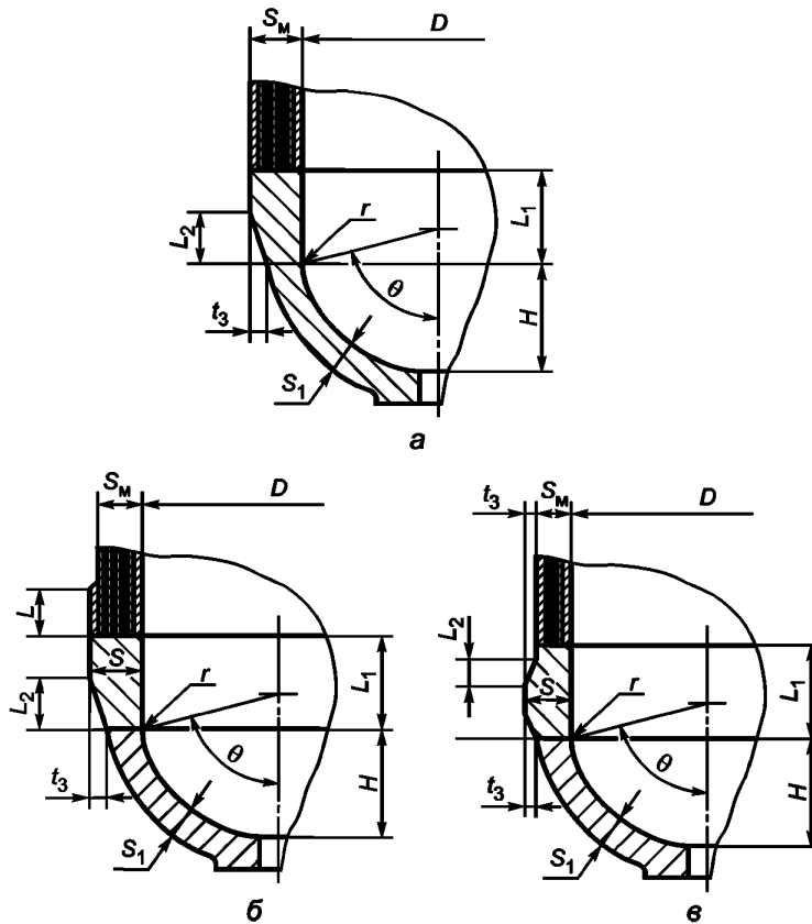
Рисунок 6.8 — Сферические днища с углом сегмента 87^\circ > \theta \geq 75^\circ , сопряженные с многослойной обечайкой посредством вставки
