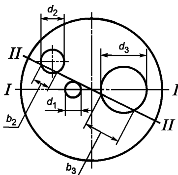
Рисунок 6.4 — Наиболее ослабленные диаметрально сечения днища
