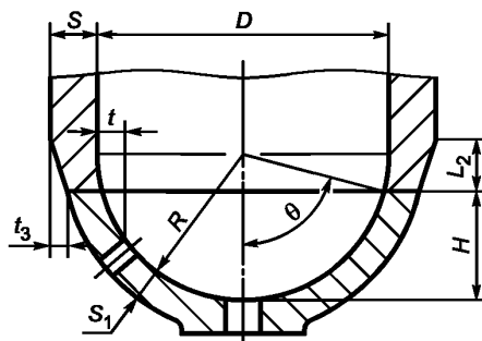
Рисунок 6.5 — Сферическое днище
