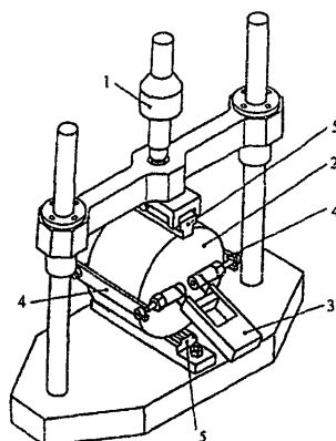
1 – нагружающее устройство; 2 – образец; 3 – тензомер; 4 – деформационные полосы; 5 – нагружающие полосы
