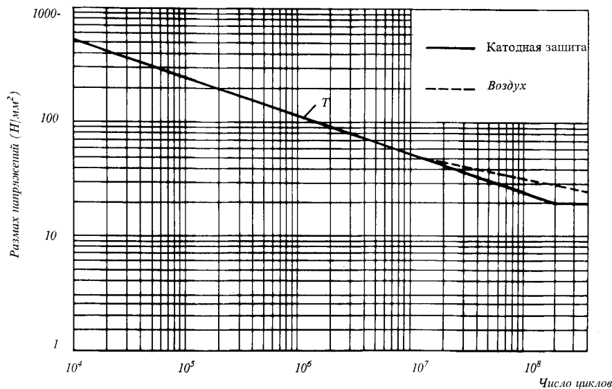
Рис. 2.4.4.8-2 Кривые S-N для трубчатых соединений
