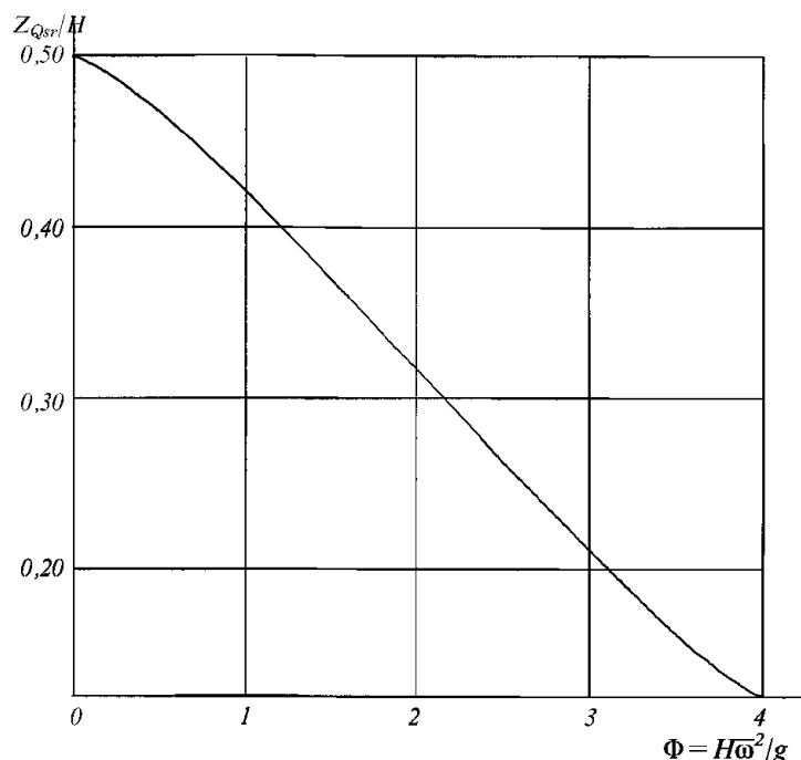
Рис. 3.1.4.13-2 Зависимость Z_{Qsr}/H от параметра \Phi = H\omega^2/g
