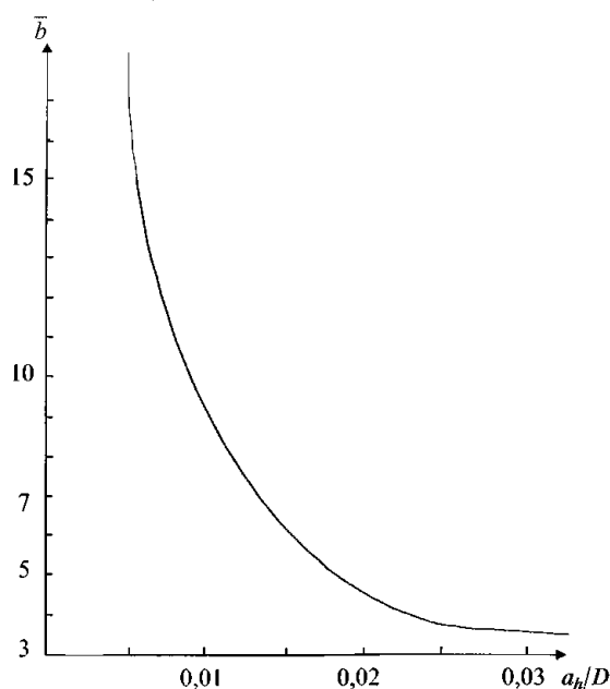
Рис. 3.3.2.3.5-1 Зависимость параметра \bar{b} от отношения a_h/D
