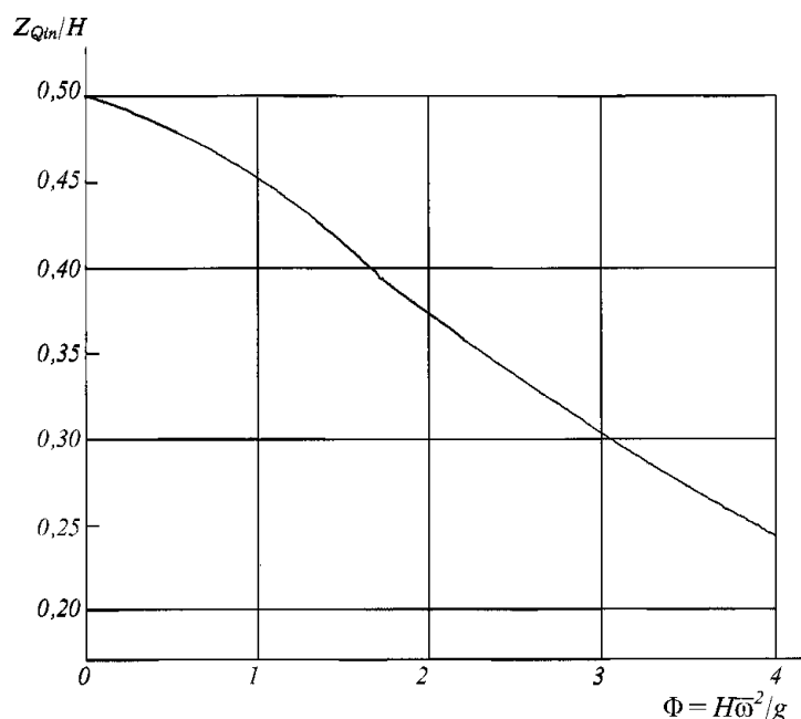
Рис. 3.1.4.13-3 Зависимость Z_{Qin}/H от параметра \Phi = H\omega^2/g
