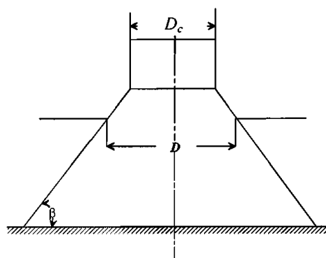
Рис. 3.3.2.3.5-3 Коническая преграда
