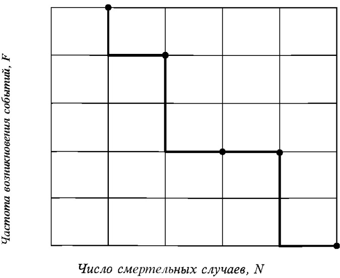
Рис. 1 Частота смертельных случаев на платформах, на которых погибло не менее N человек
