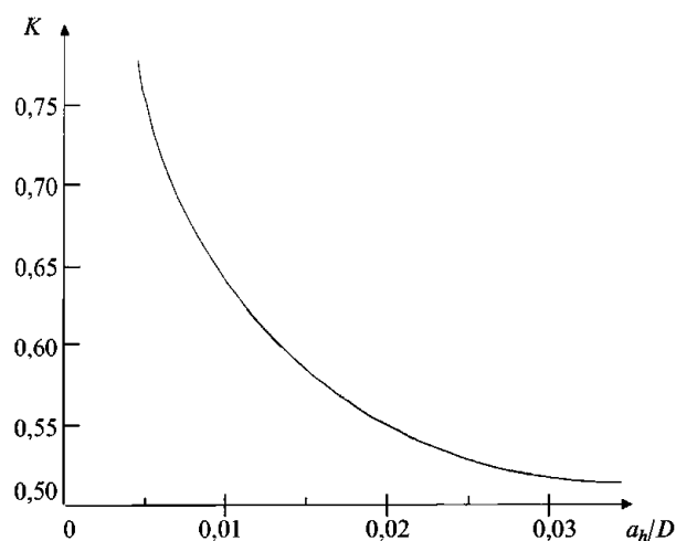
Рис. 3.3.2.3.5-2 Зависимость параметра формы K от отношения a_h/D
