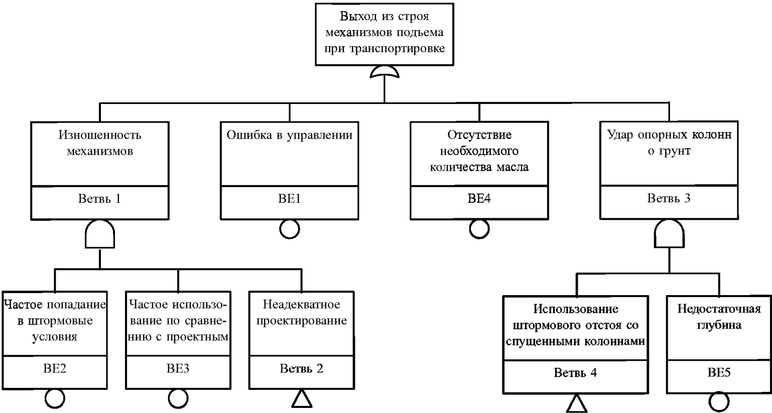
Начальное построение дерева ошибок и неполадок
