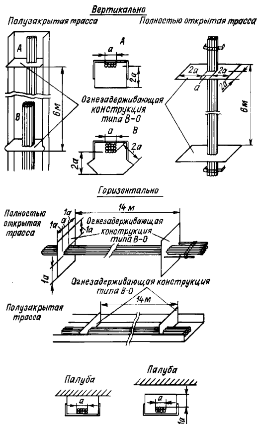
Рис. 16.8.4.3.2-2 Защита кабельных трасс огнезадерживающими конструкциями типа В-0
