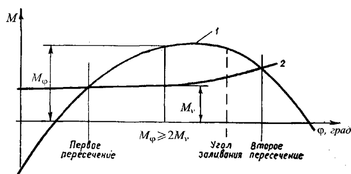
Рис. 2.6.2.1.4 Кривые восстанавливающего момента (1) и ветрового кренящего момента (2)
