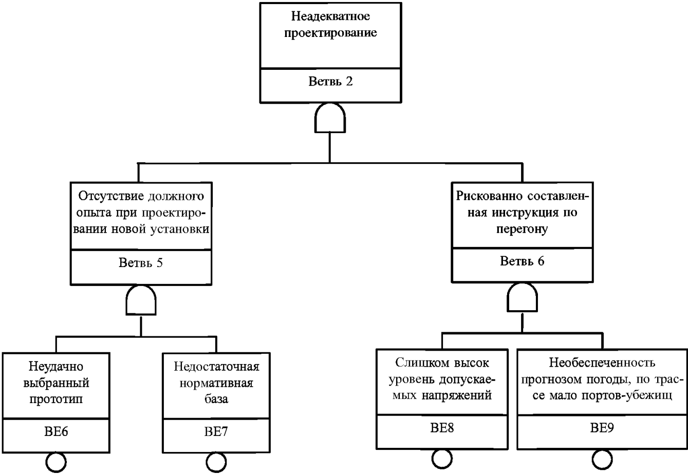
Продолжение построения дерева ошибок и неполадок
