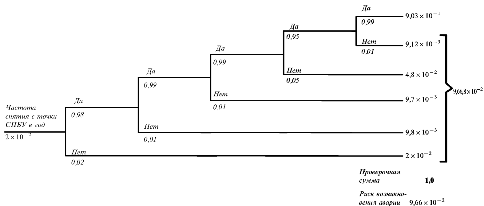
Дерево событий при транспортировках СПБУ и ППБУ
