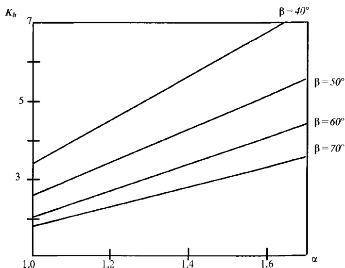
Рис. 3.3.2.3.7 Зависимость коэффициента торосистости K_h для конических опор от отношения \alpha = h_{cons}/h_{rat} и угла конусности \beta
