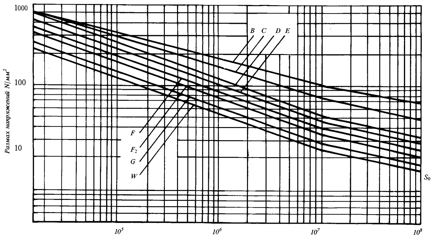
Рис. 2.4.4.8-1 Кривые усталости
