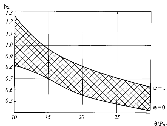
Рис. 3.1.6.1 Обобщенный коэффициент динамичности: \theta — несущая частота аксилограммы; P_{01} — низшая частота горизонтальных колебаний
