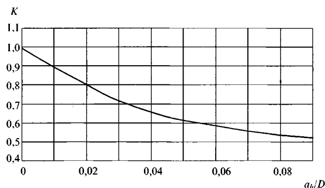
Рис. 3.3.2.3.3-1 Параметр формы K в зависимости от a_h/D
