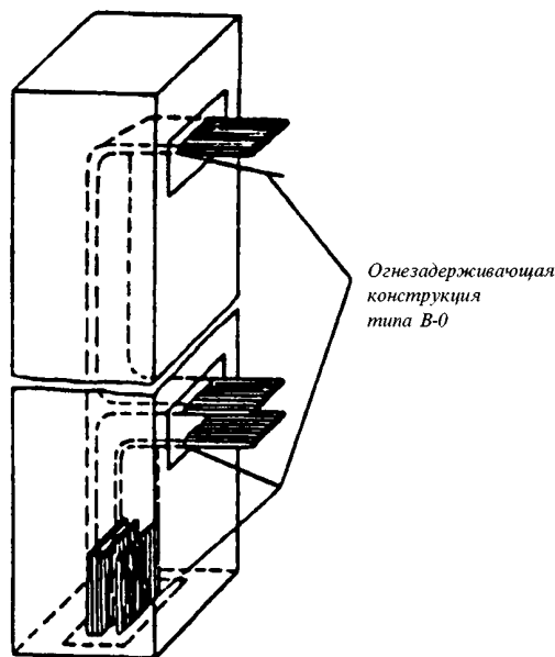
Рис. 16.8.4.3.1 Защита кабельной трассы полностью закрытой конструкцией В-0
