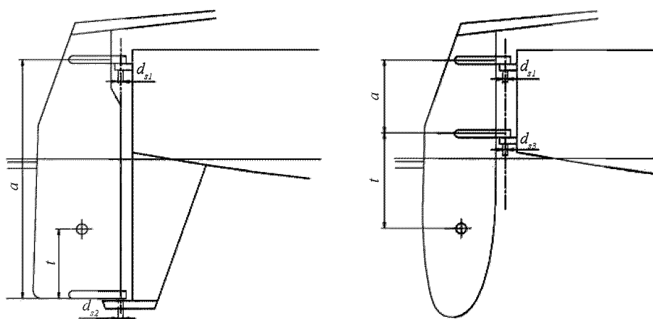
Рис. 2.5.3 Транцевые рули
