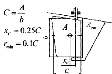
Рис. 2.2.4-3 Руль с подпятником и большим skeгом
