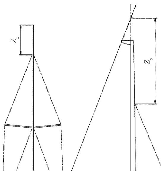
Рис. 5.4.1.6 Размеры топа мачты
