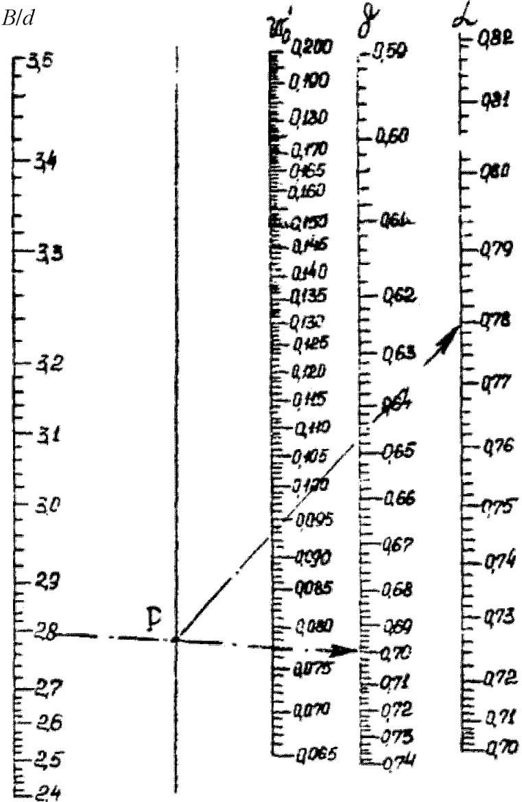
Рис. 3-4 Номограмма для определения приведенного коэффициента демпфирования, \omega'_0 , для судов с большим коэффициентом общей полноты
