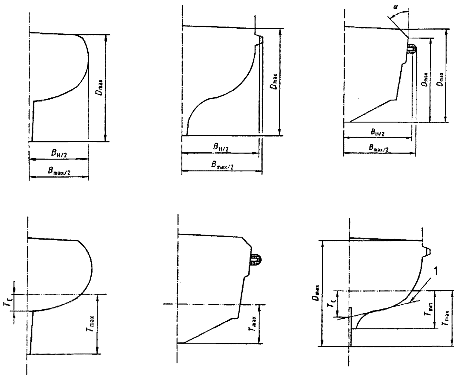
Рис. 3.2.7 Определение размеров B_{\max} , B_H , D и T(d)
