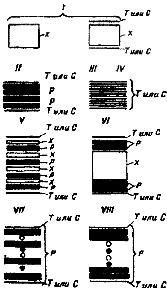
Рис. 6.1.1 Схемы армирования
