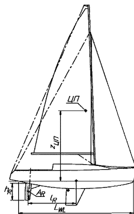
Рис. 3.1.2 Элементы парусного судна
