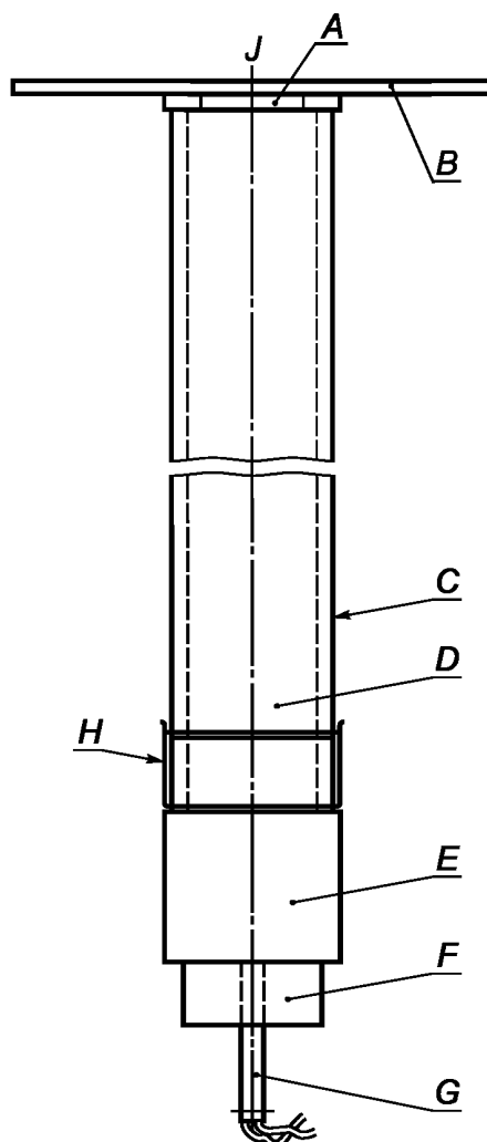
А — прокладки; В — контрольная пластина; С — стальная трубка; D — испытуемая химическая продукция; E — бустер, состоящий из циклотриметилентринитрамина/парафина или ТЭН/тринитротолуола; F — держатель детонатора; G — детонатор; H — пластмассовая мембрана; J — датчик скорости
