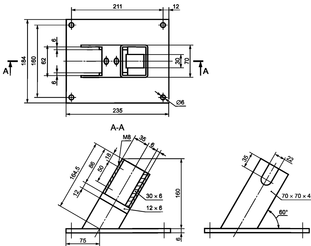
Рисунок 5 — Опорный стенд
