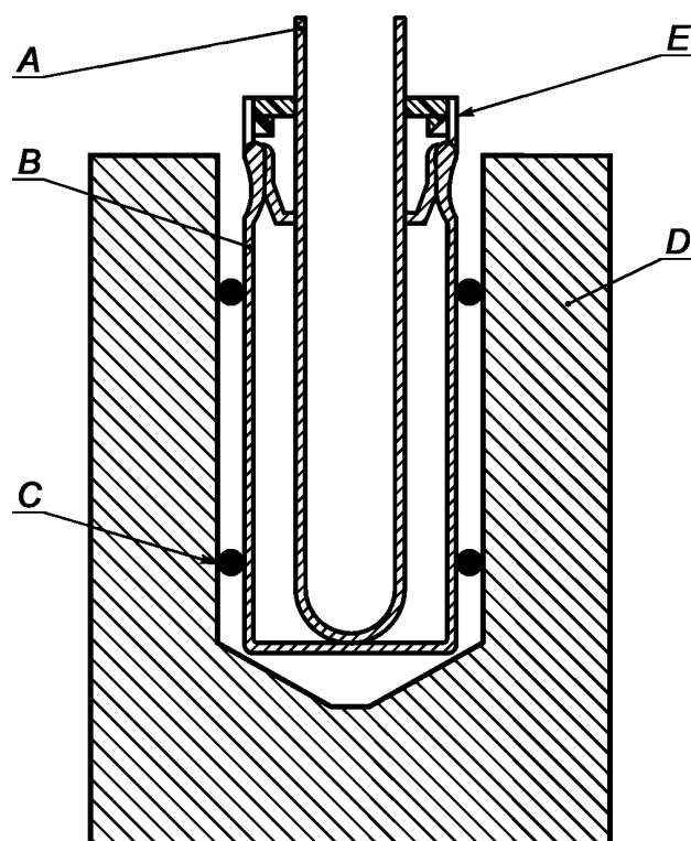
А — стеклянная трубка; В — стеклянный флакон (12 мл в комплекте А, 16 мл в комплекте В); С — О-видное кольцо (только в комплекте А); D — свинцовый блок; E — пробка
