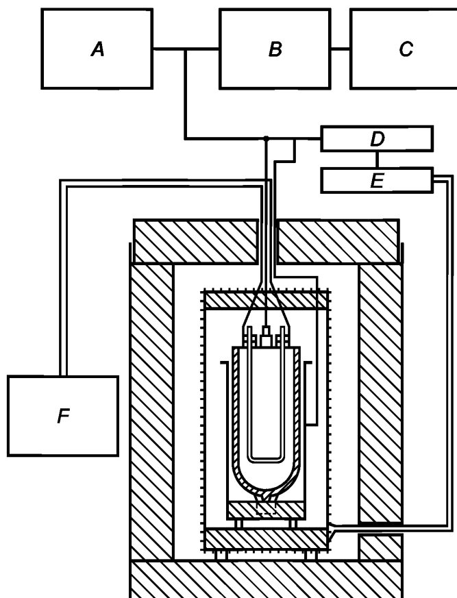
A — многоточечный регистратор и регулятор температуры (10 мВ); B — наружная установка на ноль; C — записывающее устройство высокой точности; D — управление; E — реле; F — внутренний первичный нагреватель
