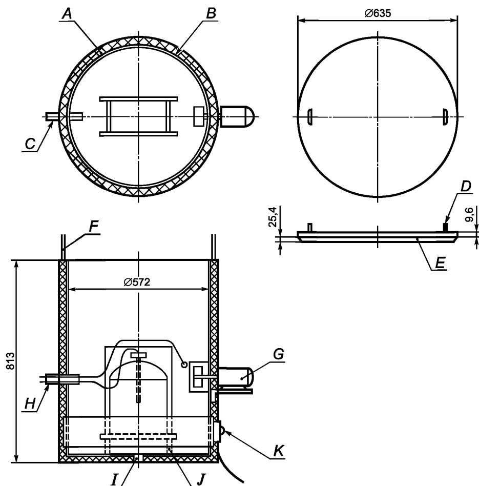
A — изоляция толщиной 25 мм; B — барабан без дна, 220 л; C — труба, 19 мм; D — стержень с петлей, 9,6 мм; E — изоляция на стальном покрытии; F — контрольный кабель, 3 мм; G — вентилятор; H — термометры и контрольные приборы; I — дренаж; J — угловая стойка, 25 мм; K — нагреватель барабана, 2 кВт
