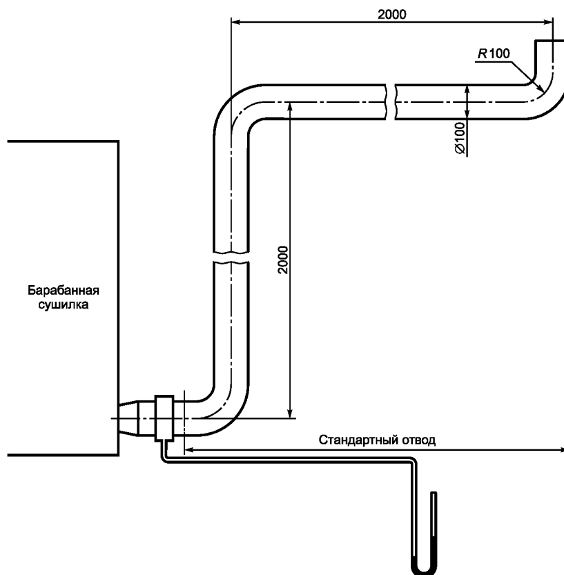
Рисунок А.2 — Стандартный отвод
