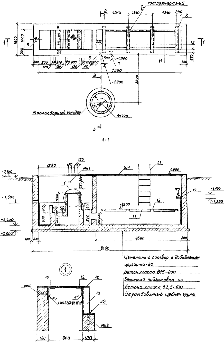
Схема расположения элементов грязеотстойника и маслобенного колодца
