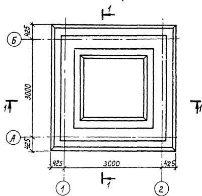
План днища
