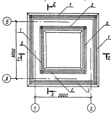
Схема расположения каркасов
