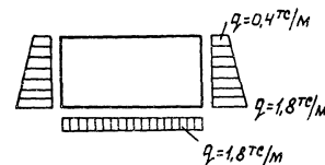
Схема расчетных нагрузок
