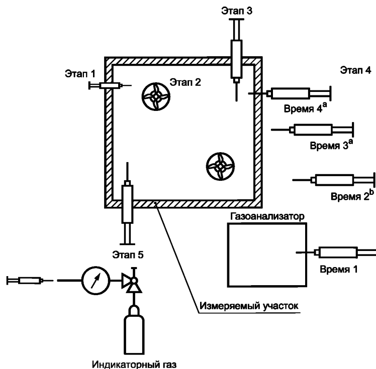
Рисунок 1 — Общая схема метода установки и этапов снижения концентрации индикаторного газа
