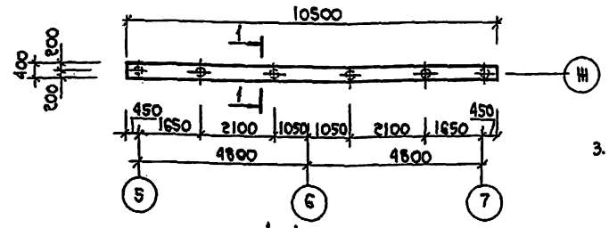
План ростверка под брандмауэрную стену
