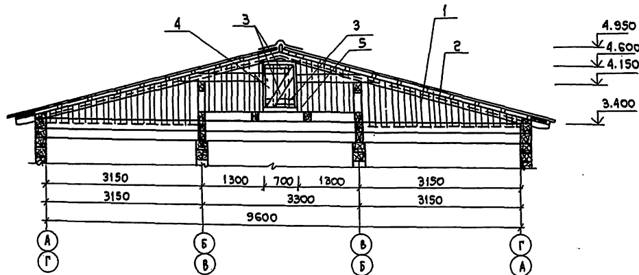
Фронтон по оси 1(19)
