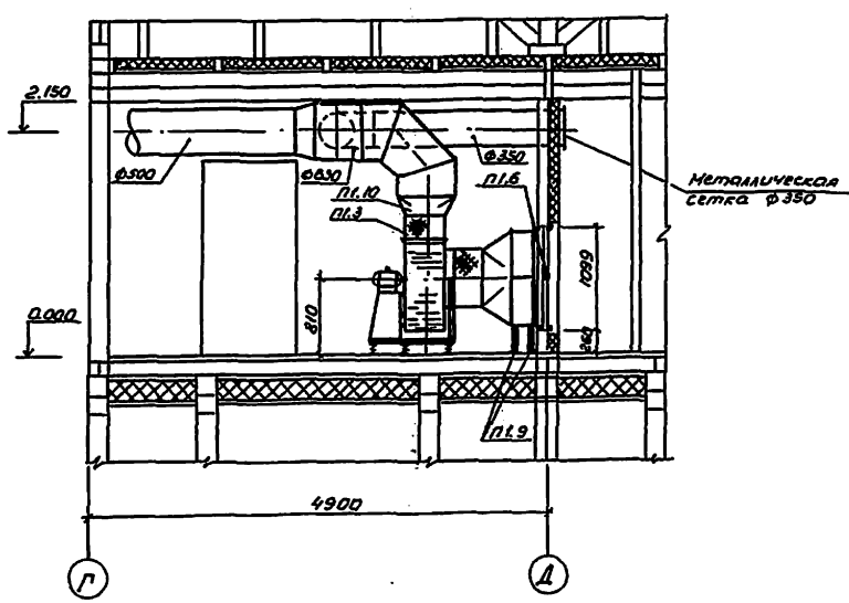
разрез 2-2
