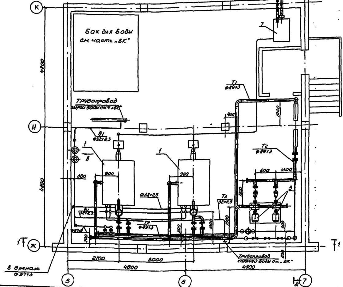
План на отвн. 0.000
