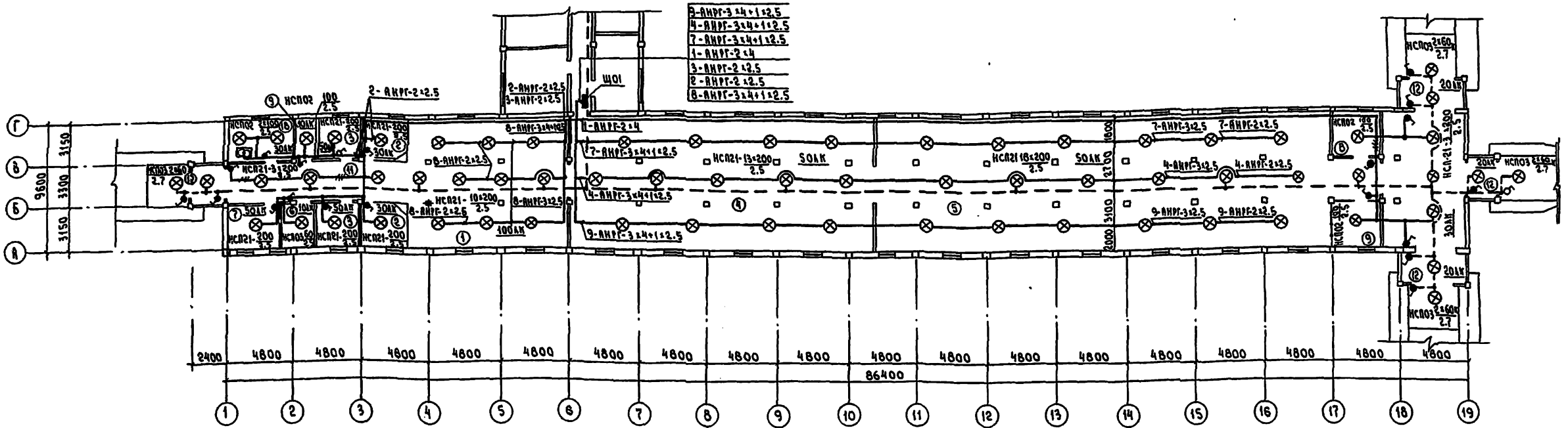
РАСЧЕТНАЯ СХЕМА ОСВЕТИТЕЛЬНОЙ СЕТИ УОИ
