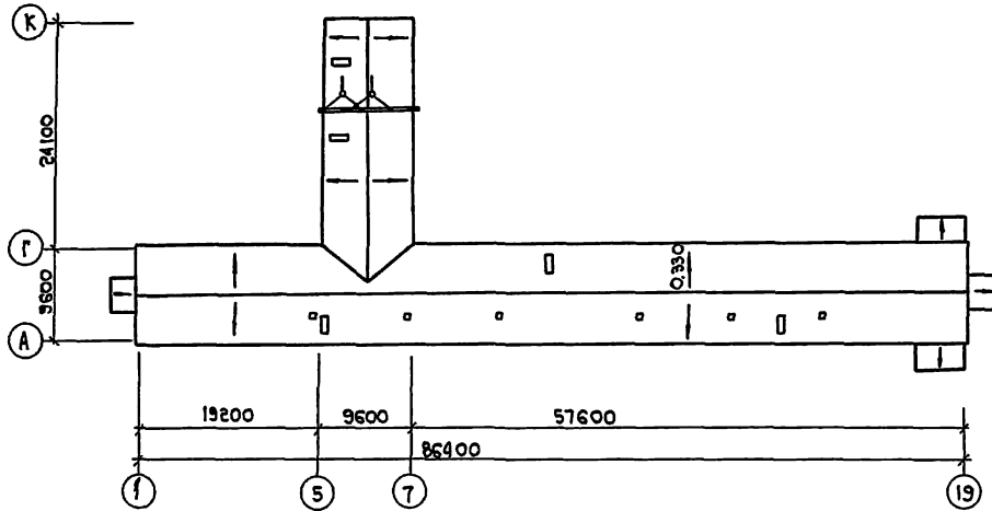
План кровли
