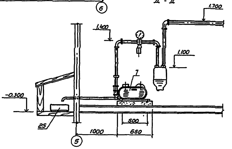
Схема разводки вакуумпробод.
