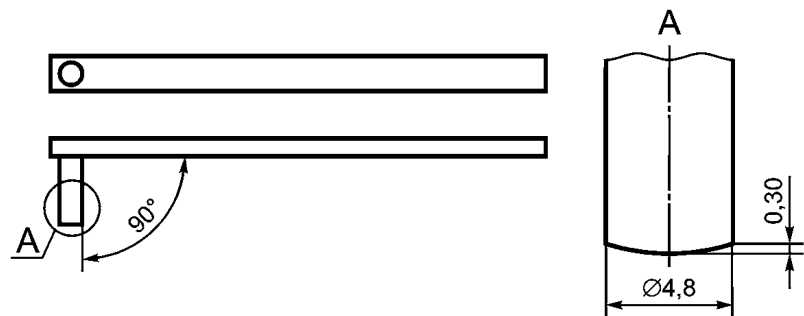
А — Скругленный контактный наконечник
