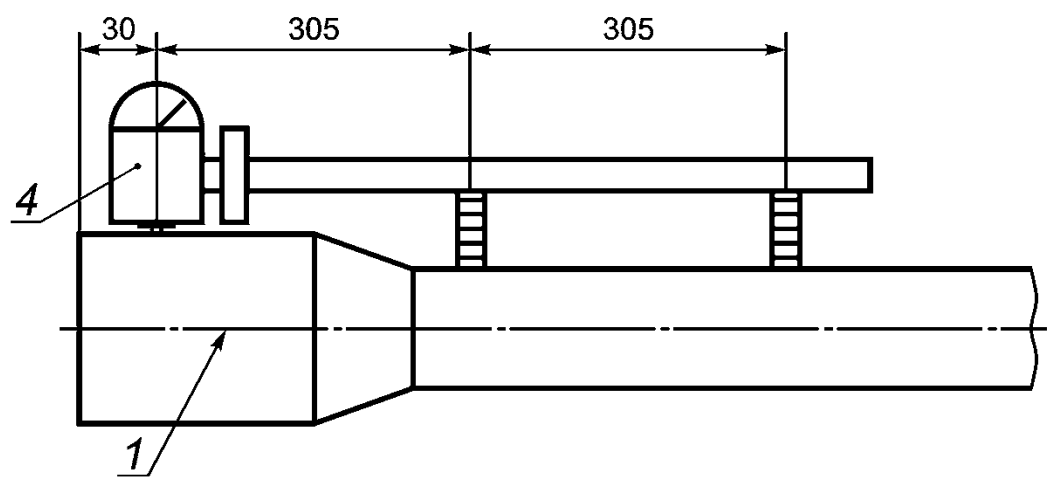
a — Измерение соосности высадки и тела трубы
