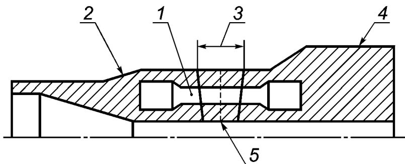
а — Расположение образца для испытания на растяжение
