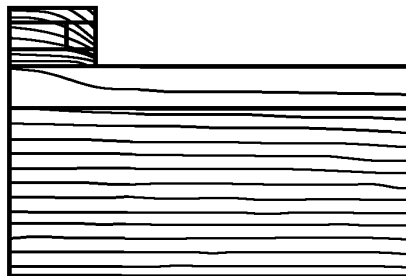
Рисунок 4 — Изотермы ( \delta\theta = 0,05^\circ\text{C} ) для установленного на стене тепломера, обшитого и защищенного (цилиндрическое сечение)
