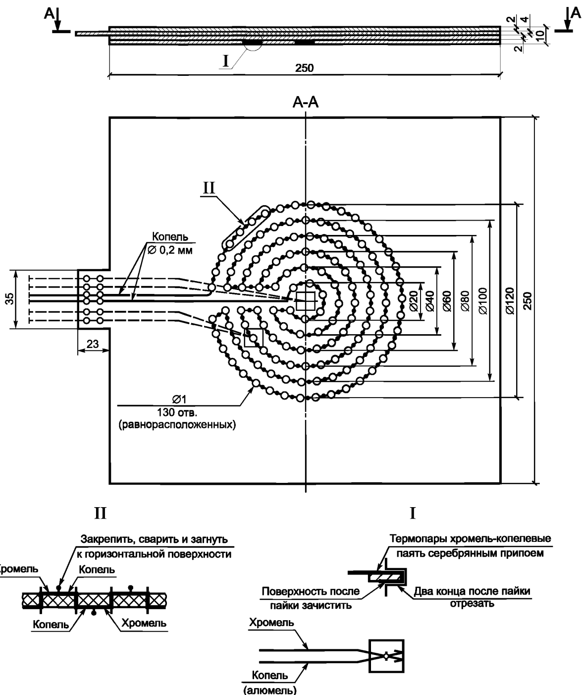
Рисунок 2 — Пример исполнения тепломера и закрепленных на нем термодатчиков
