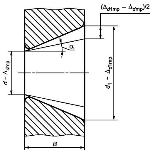
Рисунок 5 — Действительное коническое отверстие
