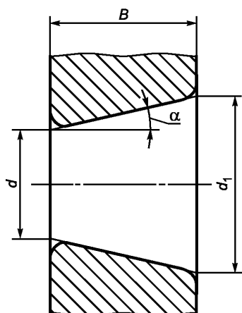
Рисунок 4 — Номинальное коническое отверстие
