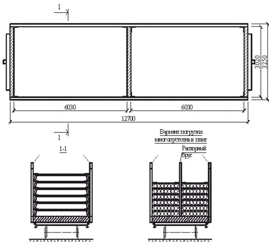
Рисунок 2 – Схема контейнера для перевозки плит
