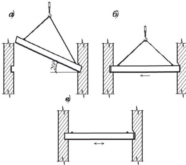
а) заведение одного конца плиты в увеличенную штрабу; б) переводение плиты в горизонтальное положение; в) контроль симметричного опирания плиты
