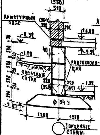
1-1 для стены \delta=510 (550)
