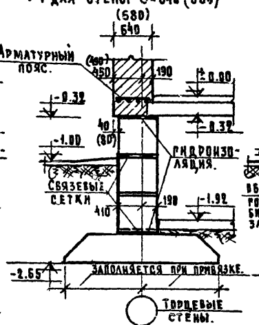
1-1 для стены \delta=640 (680)
