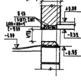
17-17 ДЕТАЛЬ ОКОННОГО ПРОЕМА ДЛЯ СТЕНЫ С ОБЩЕДОМНЫМ КИРПИЧОМ ( 640; 680 ) 510; 550
