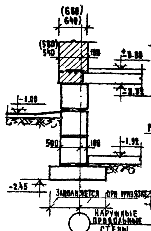
3-3 для стены \delta=640 (680)
