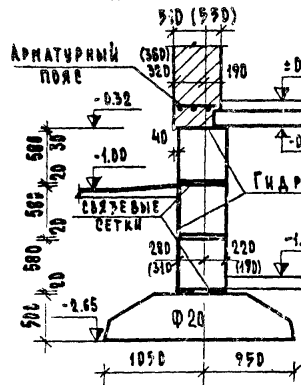
14-14 ДАД СТЕНЫ \delta=510 ( >50 )
