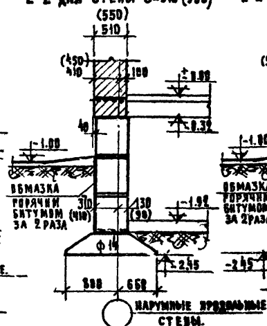
2-2 для стены \delta=510 (550)
