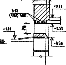
17-17 ДЕТАЛЬ ОКОННОГО ПРОЕМА ДЛЯ СТЕНЫ ИЗ ПИАНТЕАДОГО КИРПИЧА ( 640; 680 ) 510; 550
