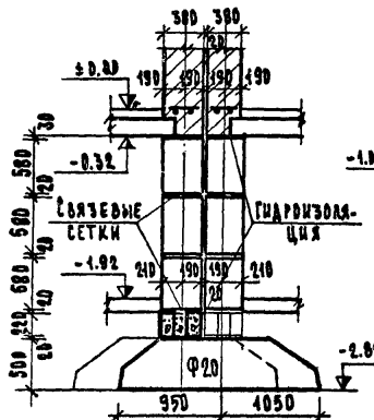
РАЗРЕЗ V-V
