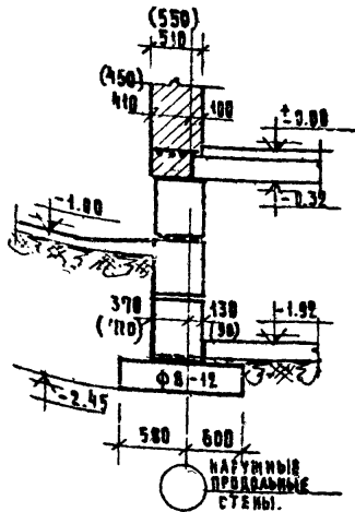
3-3 для стены \delta=510 (550)
