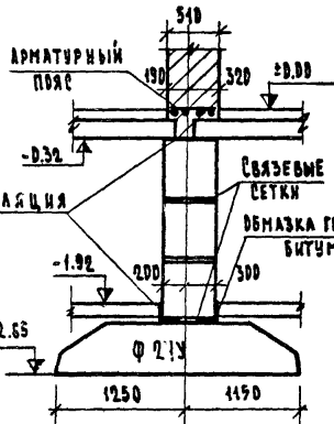
РАЗРЕЗ V-V
