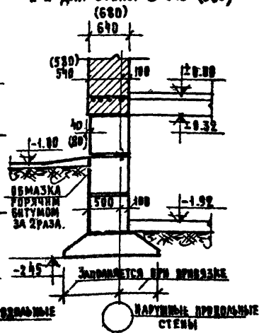
2-2 для стены \delta=640 (680)
