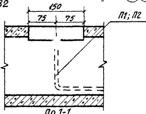
Деталь "А" ПО 1-1
