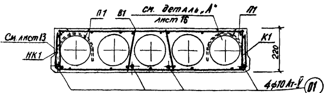
Разрез 1-1
