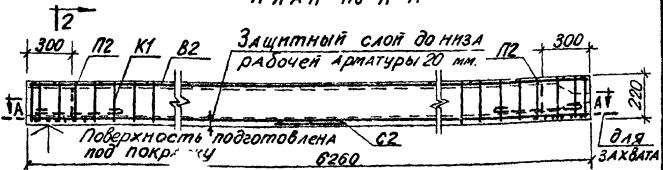
Разрез 1-1
