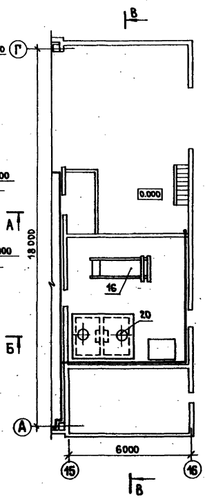
ПЛАН НА ОТМ. 0.000
