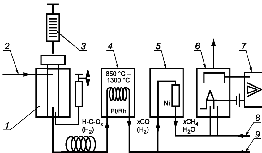
1 — капиллярная колонка; 2 — газ-носитель ( +H_2 + nC_5 , если обозначено); 3 — образец C_nH_mO_x ; 4 — реактор разложения; 5 — реактор гидрогенизации (метанайзер); 6 — FID; 7 — электрометр; 8 — воздух; 9 — водород
