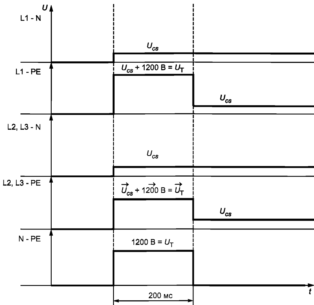
S1 — главный выключатель; S2 — таймер, замыкающийся через 200 мс после главного выключателя; F1 — максимальная сверхтоковая защита, заявленная изготовителем; F2 — плавкий предохранитель для защиты трансформатора ВПН (должен выдержать 300 А в течение 200 мс); T1 — трансформатор источника питания с напряжением на вторичной обмотке U_{cs} ; T2 — трансформатор ВПН с напряжением на первичной обмотке U_{cs} , на вторичной — 1200 В; R1 — токоограничивающий резистор для регулирования тока короткого замыкания на источнике питания при U_{cs} ; R2 — токоограничивающий резистор для регулирования тока короткого замыкания в цепи ВПН до 300 А (приблизительно 4 Ом); УЗИП — испытуемое устройство
