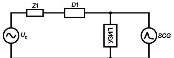
Рисунок 6а — Цепь для испытания УЗИП с сопровождающим током I_{fi} ниже заявленной способности выдерживать ток короткого замыкания
