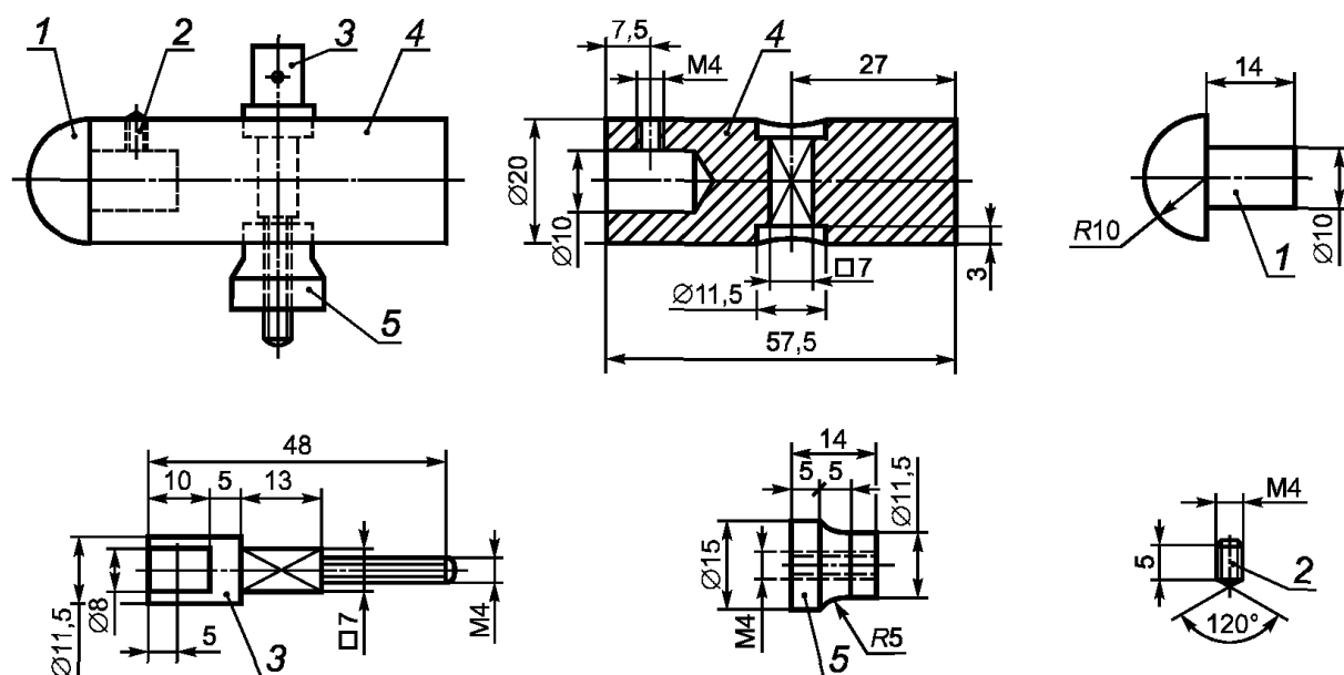
Рисунок 10а — Испытательная установка
