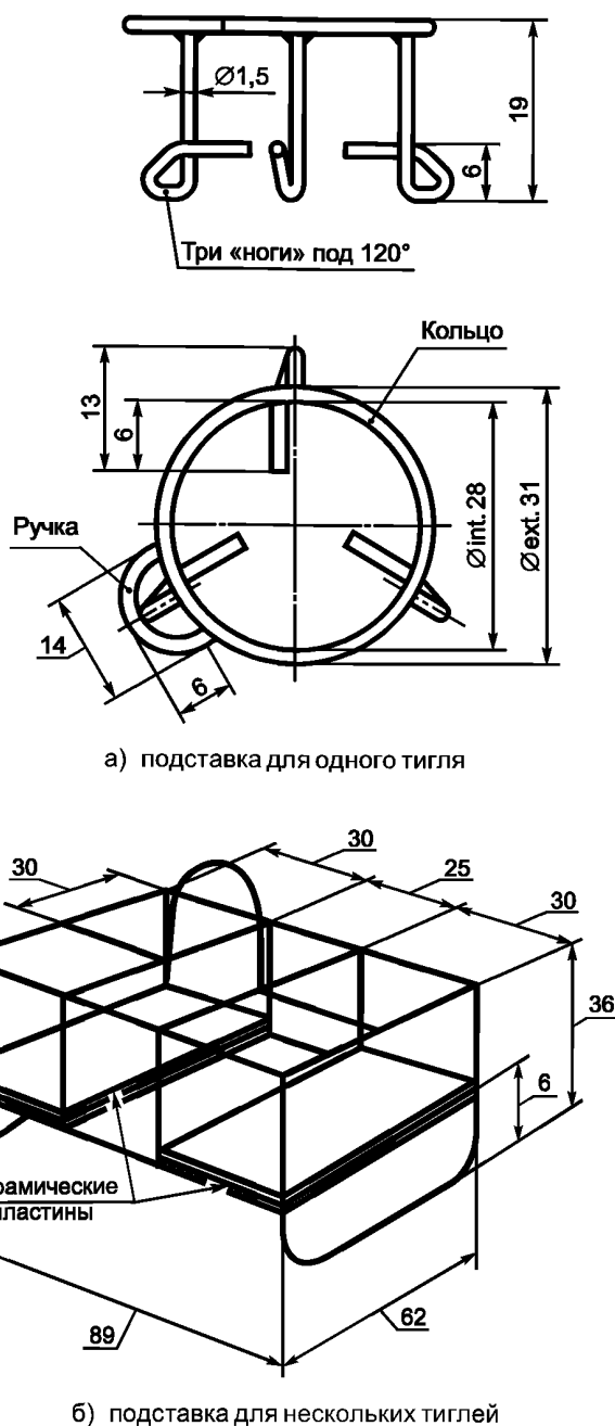
Рисунок 3 — Подставки для тиглей из термостойкой проволоки (размеры даны в миллиметрах)
