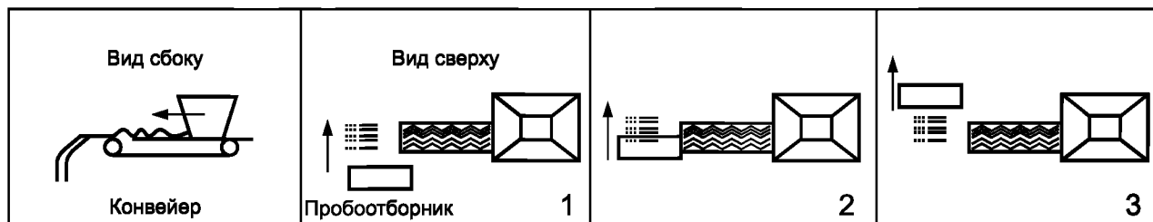
Рисунок Ж.1 — Схематичное изображение отбора пробы на перепаде потока
