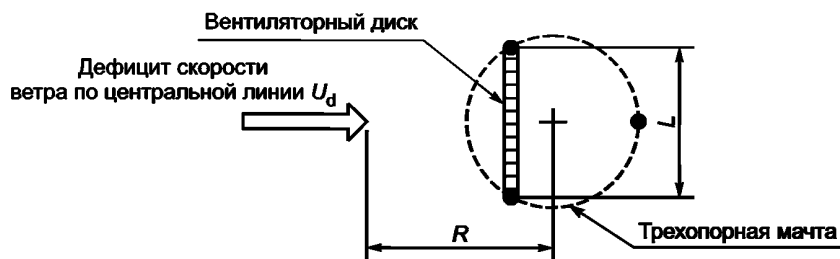
Рисунок G.7 — Представление трехопорной решетчатой мачты с указанием дефицита скорости ветра по центральной линии; представление вентиляторного диска мачты с шириной фронтальной поверхности L и расстоянием R от центра мачты до точки наблюдения
