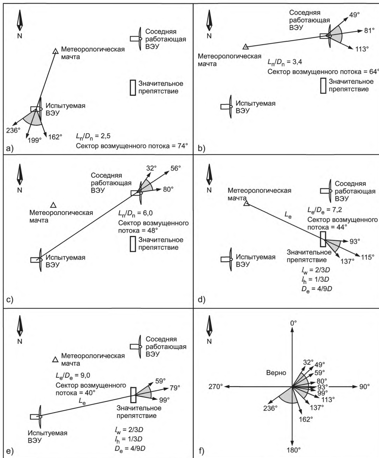
Рисунок А.2 — Пример секторов, которые необходимо исключить из-за воздействия турбулентного следа на испытываемую ВЭУ в результате влияния соседней работающей ВЭУ и значительного аэродинамического препятствия
