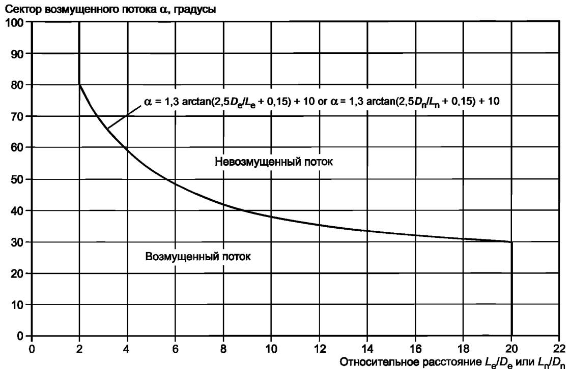
Рисунок А.1 — Секторы, которые необходимо исключить из-за возмущенного воздушного потока, вызванного соседней работающей ВЭУ и значительными аэродинамическими препятствиями
