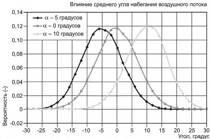
Рисунок J.6 — Распределения вероятностей для трех различных средних углов набегания воздушного потока
