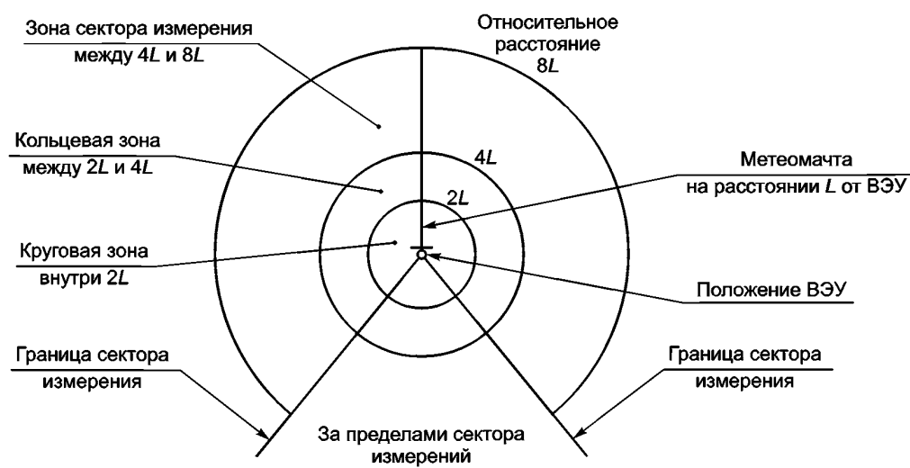
Рисунок В.1 — Изображение местности, оценку которой нужно провести, вид сверху.
