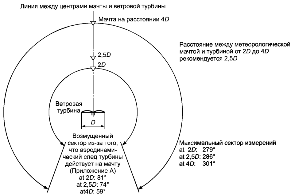
Рисунок 1 — Требования к расстоянию до метеорологической мачты и максимально допустимым секторам измерений
