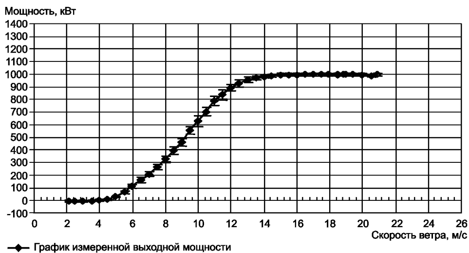
График измеренной выходной мощности с поправкой на плотность воздуха на уровне моря 1,225 \text{ кг/м}^3 (база данных В)
