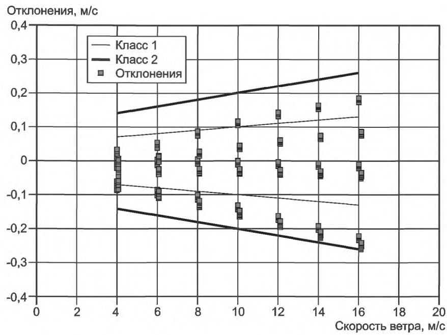
Рисунок J.9 — Пример отклонений для чашечного анемометра класса 2.0А
