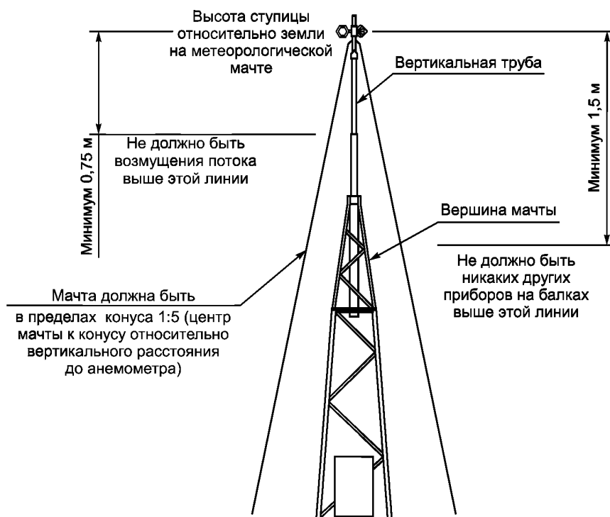
Рисунок G.1 — Пример установки анемометра в верхней части мачты и требования к монтажу
