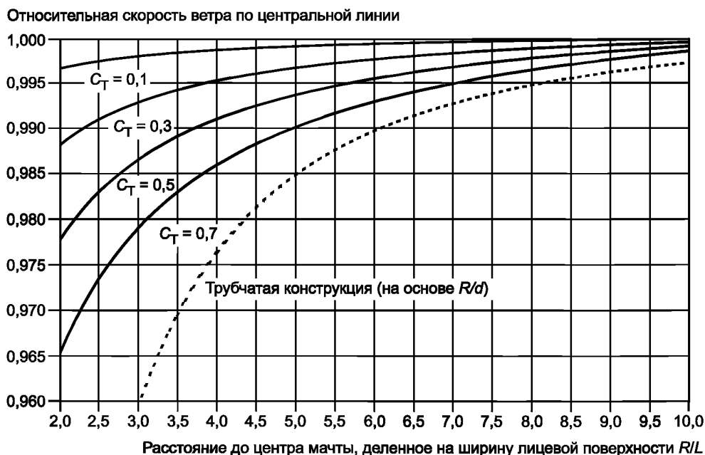
Рисунок G.9 — Относительная скорость ветра по центральной линии в функции расстояния R до центра трехопорной решетчатой мачты с шириной фронтальной поверхности L для различных значений C_T
