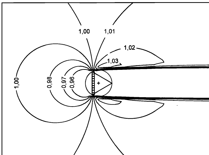
Рисунок G.8 — Поле распределения скоростей воздушного потока вокруг трехопорной решетчатой мачты с C_T = 0,5 , нормализованное полем скоростей невозмущенного воздушного потока (слева); компьютерный расчет на основе двумерных уравнений Навье — Стокса и по теории вентиляторного диска
