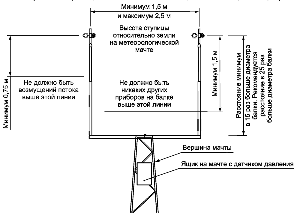
Рисунок G.2 — Пример альтернативного крепления основного и контрольного анемометров в верхней части мачты, а также флюгера и других приборов на балке
