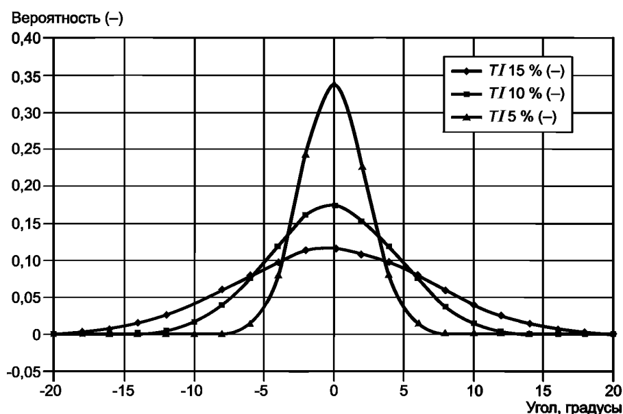
Рисунок J.4 — Распределение вертикальных составляющих скорости ветра в предположении фиксированного отношения между горизонтальным и вертикальным средними квадратическими отклонениями в скорости ветра
