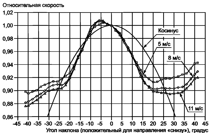
Рисунок J.1 — Измеренные угловые характеристики чашечного анемометра в сравнении с косинусной реакцией
