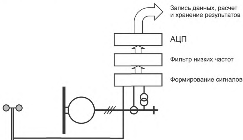
Рисунок 3 — Элементы системы измерений
