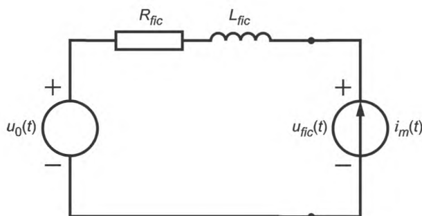
Рисунок 4 — Расчетная электрическая сеть для моделирования
