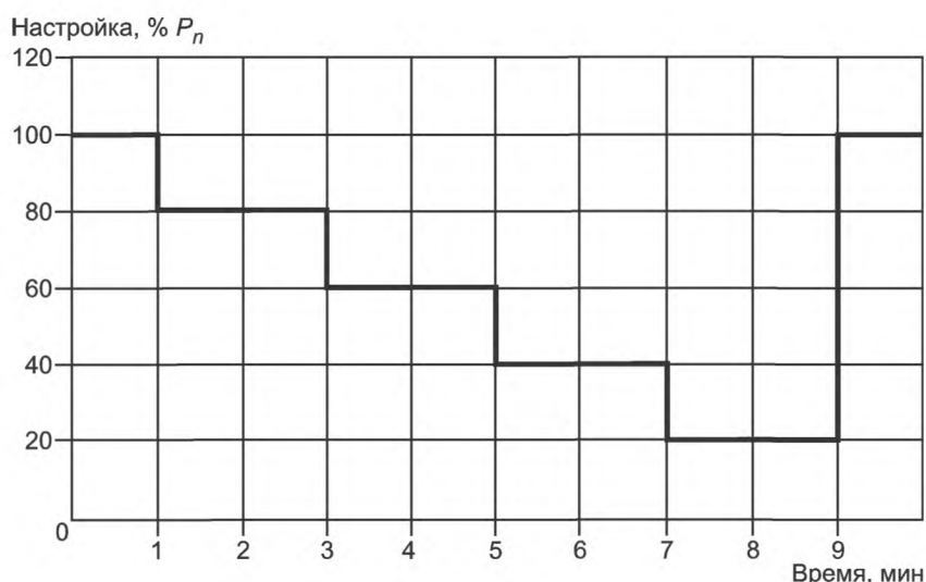
Рисунок 1 — Уставки активной мощности
