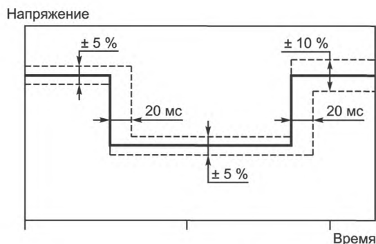
Рисунок 6 — Допустимые отклонения формы провала напряжения
