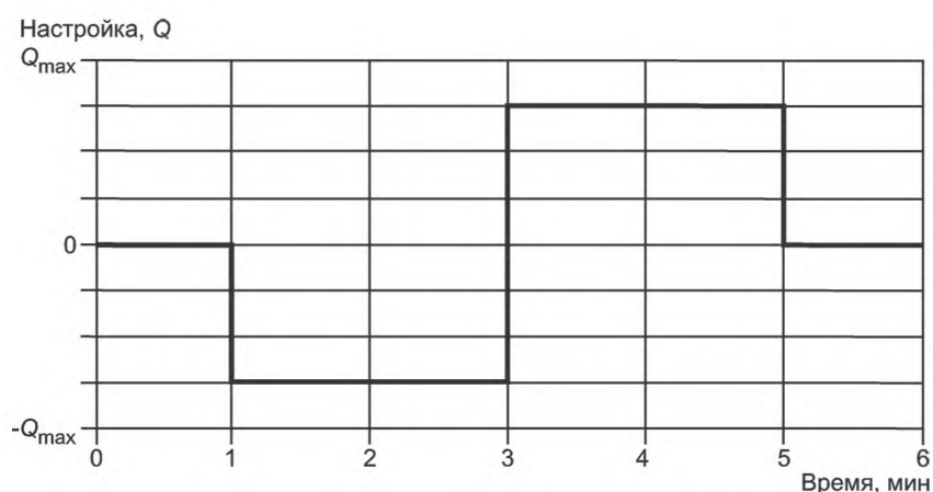
Рисунок 2 — Настройка уставки реактивной мощности
