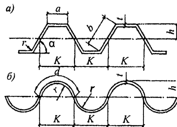
а – трапециевидный гофр; б – волнистый гофр
