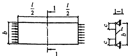
Рисунок 11 – Расчетная схема сжатого тонколистового элемента
