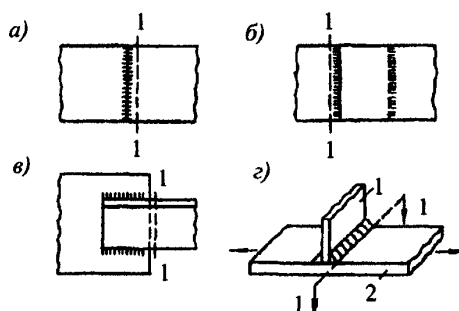
Рисунок 1 – Схемы сварных соединений конструкций
