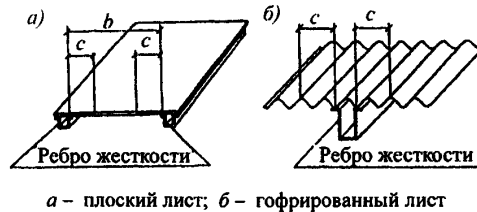
Рисунок 12 – Расчетная схема тонколистовых конструкций, усиленных продольными ребрами
