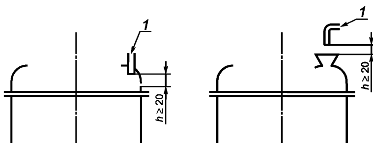
Рисунок 9 — Примеры создания «воздушного зазора»
