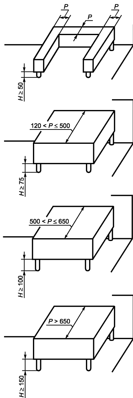
Рисунок А.12 — Подставки для машин
