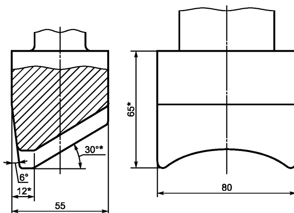
Рисунок А.2 — Замок
