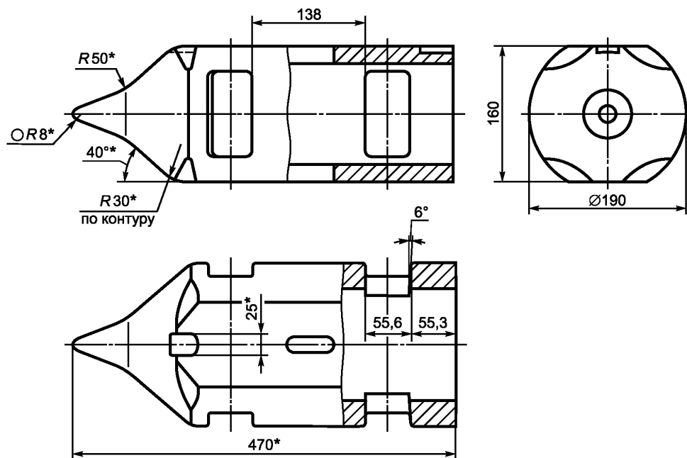
Рисунок А.3 — Направляющий элемент
