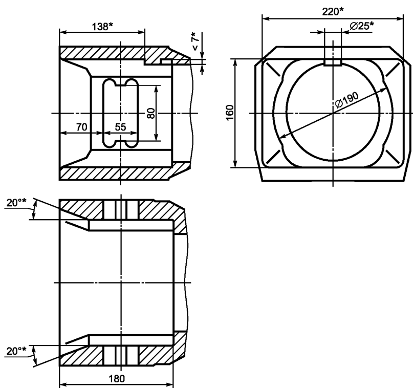
Рисунок А.1 — Корпус сцепки
