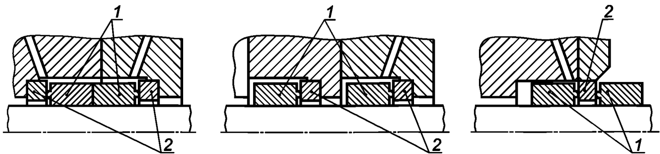
D1 — компоновка «спина к спине»
