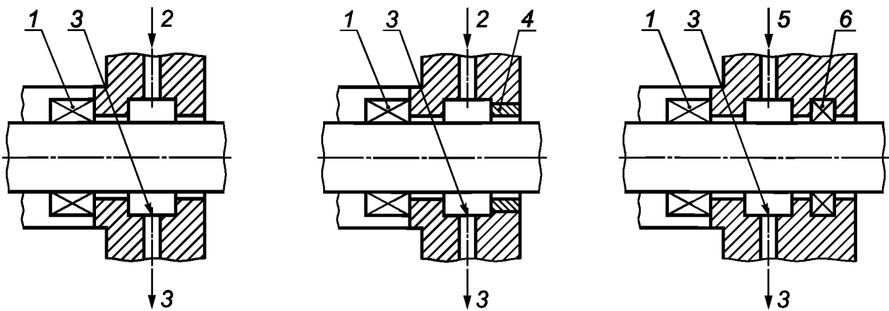
Q1 — основное уплотнение без дроссельной втулки или дополнительного уплотнения
