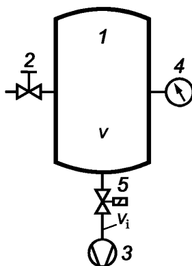
1 — измерительная камера; 2 — клапан напуска газа; 3 — испытуемый насос; 4 — вакуумметр для измерения p_{t1} , p_{t2} , p_{t3} ; 5 — быстродействующий клапан; V — объем измерительной камеры; V_i — объем соединительного трубопровода между испытуемым насосом и быстродействующим клапаном
