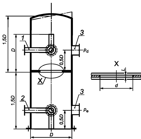
1 — патрубок напуска газа; 2 — патрубок напуска газа и точка измерения температуры T_D ; 3 — патрубок для подсоединения вакуумметра и масс-спектрометра; D — внутренний диаметр измерительной камеры, м; L — толщина стенки в диаметре отверстия, м; p_d, p_e — давления в измерительной камере, Па (или мбар)
