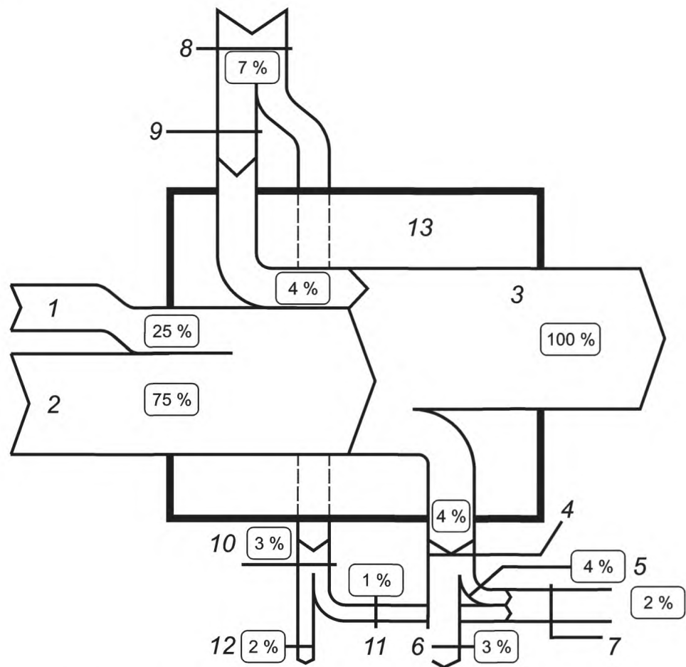
1 — энергия, расходуемая на привод ТСТ (например, электричество, топливо) E_{HW,gen,in} ; 2 — теплота окружающей среды, используемая в качестве источника тепловой энергии низкого потенциала Q_{HW,gen,in} ; 3 — теплопроизводительность (тепловая мощность) подсистемы генерации теплоты, соответствующая тепловым нагрузкам подсистем распределения теплоты Q_{HW,gen,out} = Q_{HW,dis,in} ; 4 — тепловые потери подсистемы генерации теплоты Q_{HW,gen,ls} ; 5 — тепловые потери подсистемы генерации теплоты (тепловая часть), регенерированные для отопления помещений Q_{HW,gen,ls,rbl} ; 6 — невозвратные тепловые потери подсистемы генерации (тепловая часть) Q_{HW,gen,ls,nrbl} ; 7 — общие тепловые потери подсистемы генерации, возвращаемые (рекуперированные или регенерированные) для отопления помещений Q_{HW,gen,ls,rbl,tot} ; 8 — общая дополнительная энергия подсистемы генерации теплоты W_{HW,gen,aux} ; 9 — возвращаемая дополнительная энергия подсистемы генерации Q_{HW,gen,aux,ls,rbl} ; 10 — невозвратная дополнительная энергия подсистемы генерации Q_{HW,gen,aux,ls} ; 11 — регенерированная дополнительная энергия подсистемы генерации Q_{HW,gen,aux,ls,rbl} ; 12 — нерегенерированная вспомогательная энергия подсистемы генерации Q_{HW,gen,aux,ls,nrbl} ; 13 — подсистема генерации (получения, переноса и передачи) теплоты
