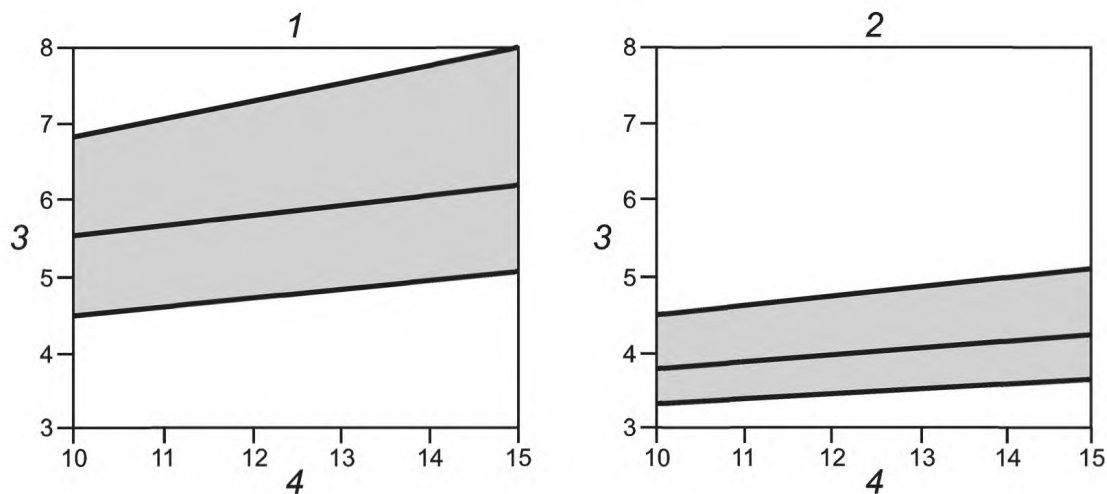
1 — температура отвода тепла \theta_{sk} = 35\text{ °C} ; 2 — температура отвода тепла \theta_{sk} = 50\text{ °C} ; 3 — K_{TP}(COP) ; 4 — температура источника тепла низкого потенциала
