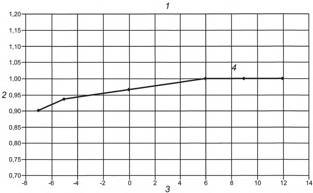
Относительная теплопроизводительность
