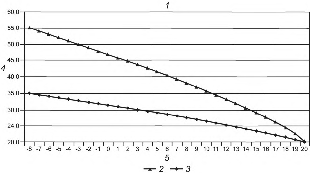
1 — температурные графики подачи теплоносителя в системы отопления; 2 — система отопления с радиаторами; 3 — напольная система отопления; 4 — подающая температура теплоносителя в систему отопления, °C; 5 — температура наружного воздуха, °C
