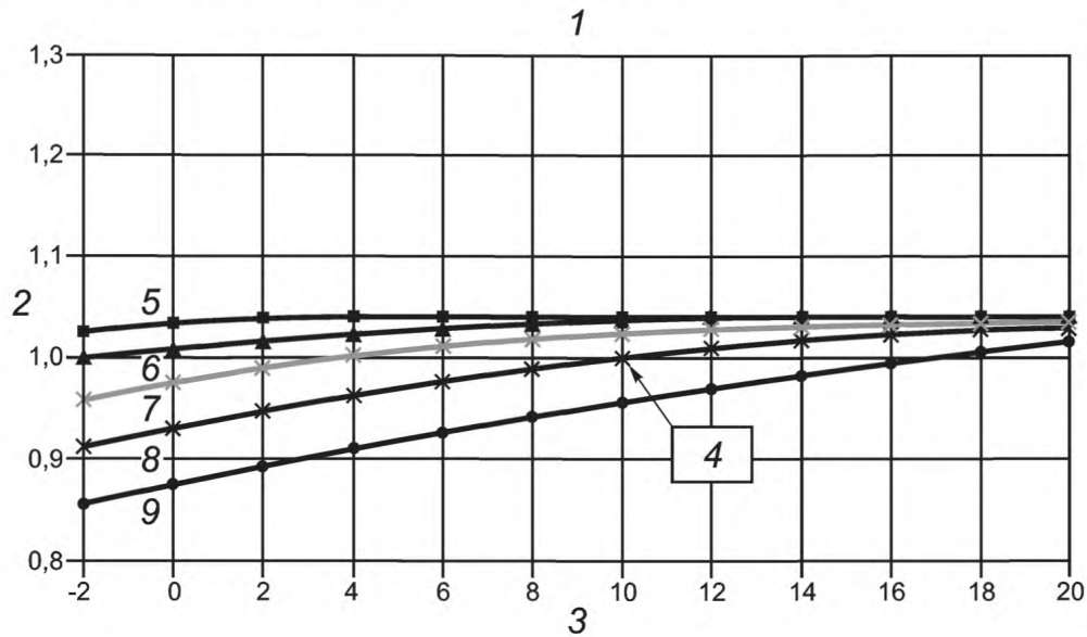
Относительная теплопроизводительность и относительный K_{\text{ТР}}(COP)
