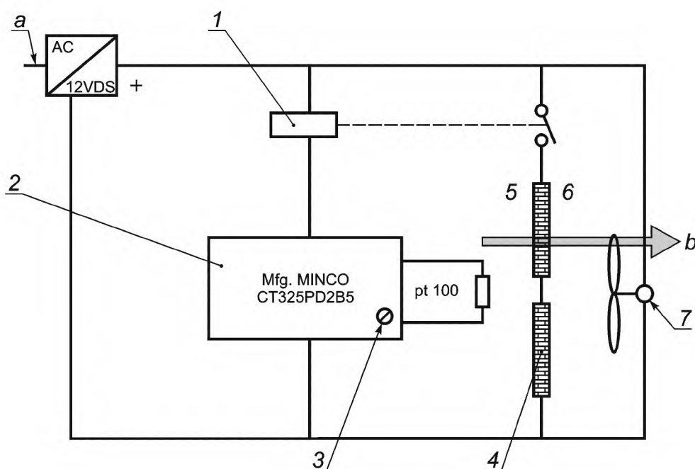
1 — реле; 2 — релейный регулятор; 3 — уставка; 4 — элемент Пельтье; 5 — холодная сторона; 6 — теплая сторона; 7 — вентилятор; a — провод с напряжением 220 В; b — направление теплового потока
