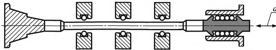
Рисунок 8 — Бурильная труба. Испытание по определению толкающего/тянущего усилия
