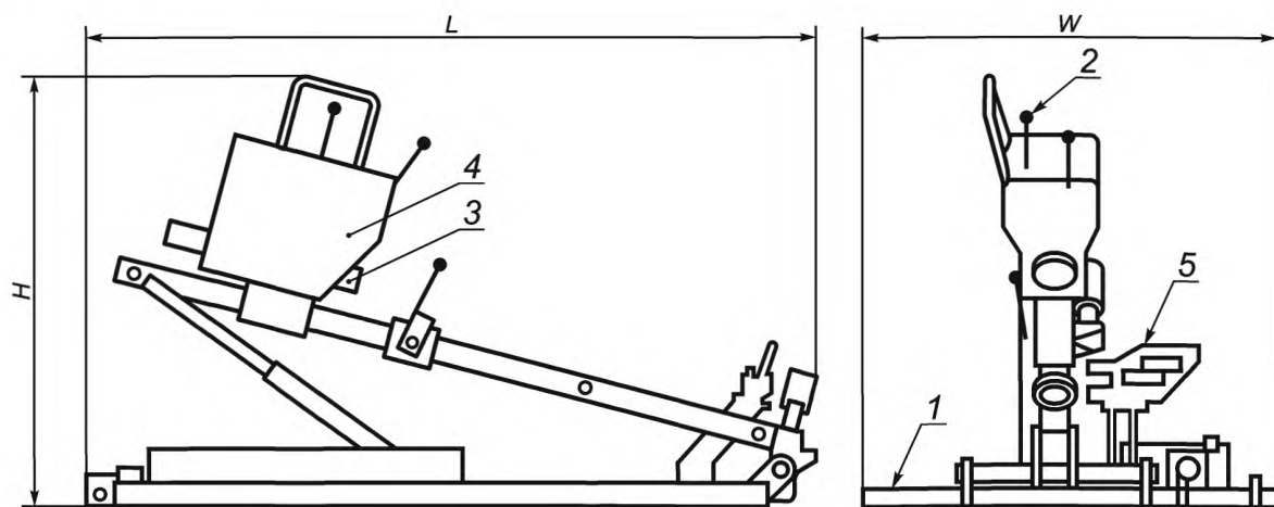
H — общая высота машины; L — общая длина машины; W — общая ширина машины; 1 — место оператора; 2 — управление процессом бурения; 3 — шпиндель; 4 — каретка; 5 — зажим
