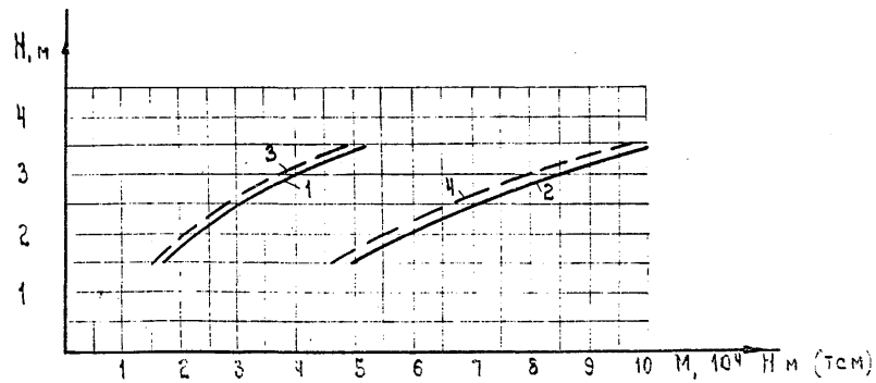
График моментов для подбора арматуры в сваях береговых опор типа 1
