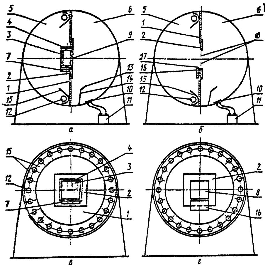
Схема диффузметра
