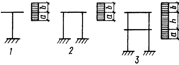
Рис. 6. 1 — одностоечная одноярусная эстакада; 2 — двухстоечная одноярусная эстакада; 3 — двухстоечная двухъярусная эстакада; h — расстояние между отметками верхних граней траверс нижнего и верхнего ярусов; a и b — высота ветровой полосы
