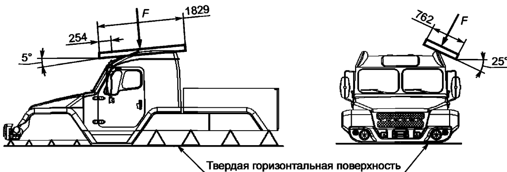
Рисунок 1 — Схема испытания защитных свойств кузова/кабины
