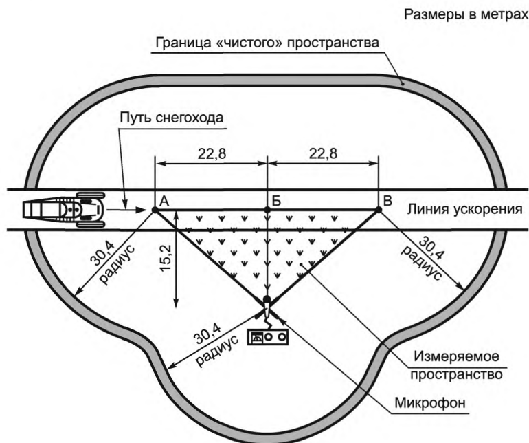
Рисунок 5 — Схема измерительного участка для определения внешнего шума
