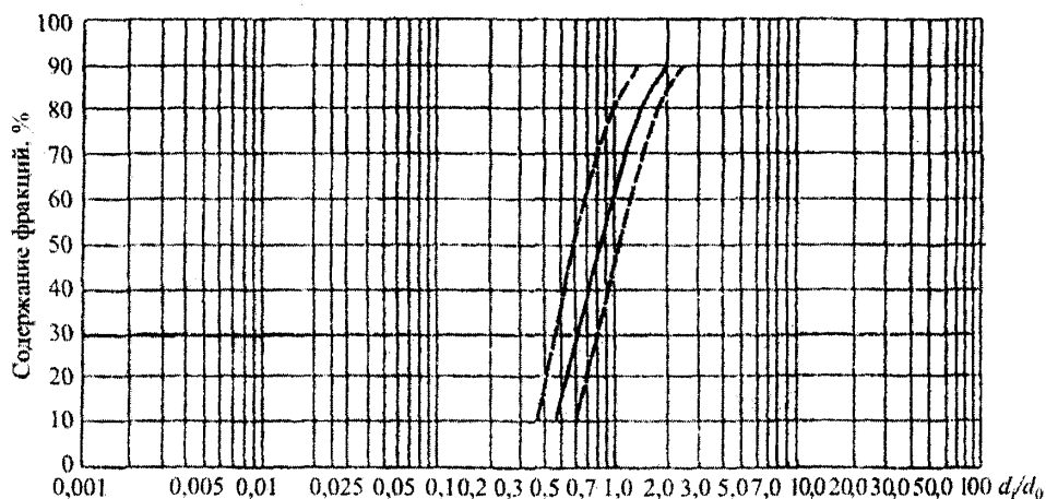
Рисунок Е.1 – График зависимости \alpha = f\left(\frac{d_i}{d_0}\right) для однородных песчаных плотин
