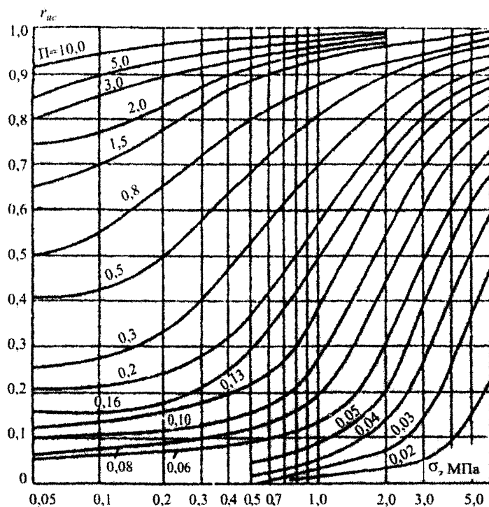
Рисунок А.1 – Номограмма для определения порового давления r_{ur}
