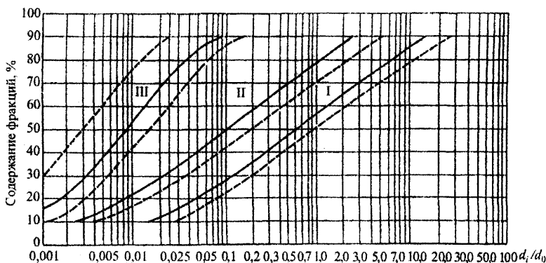
Рисунок Е.5 – График зависимости \alpha = f\left(\frac{d_1}{d_0}\right) для гравийных плотин с ядром высотой > 30 м
