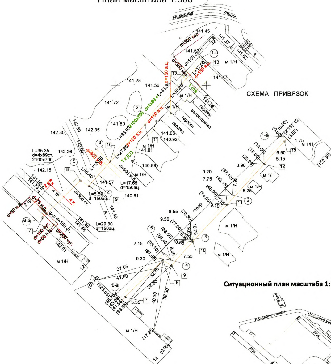
План масштаба 1:500
