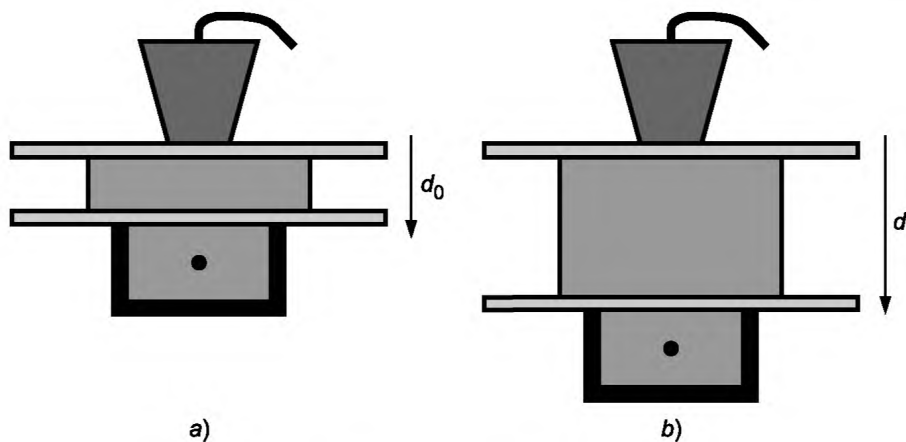
Рисунок 2 — Схема конструкции тест-объекта с термоэлементом
