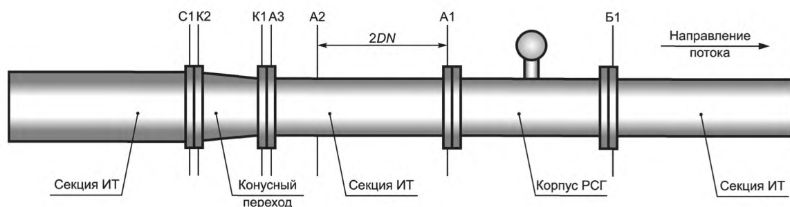
Рисунок 6 — Сечения, в которых измеряют внутренний диаметр ИТ в случае применения конусных переходов
