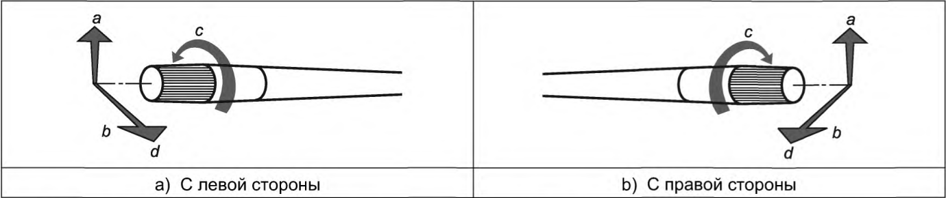
П р и м е ч а н и е — Стрелки показывают направление движения для включения/увеличения (кроме сигнала поворота). a Подъем рычага. В Японии стереотип относительно опускания, а не подъема очень слабый. b Стереотип в Японии очень слабый. c Вращение верхней части. d Передвигание.
