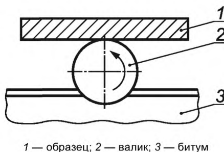
Рисунок А.1 — Нанесение горячего битума на лицевую грань образца
