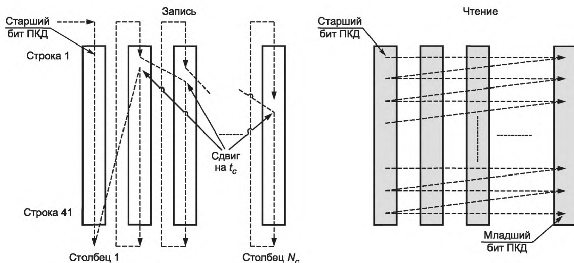
Рисунок 4 — Процедура битового перемежения
