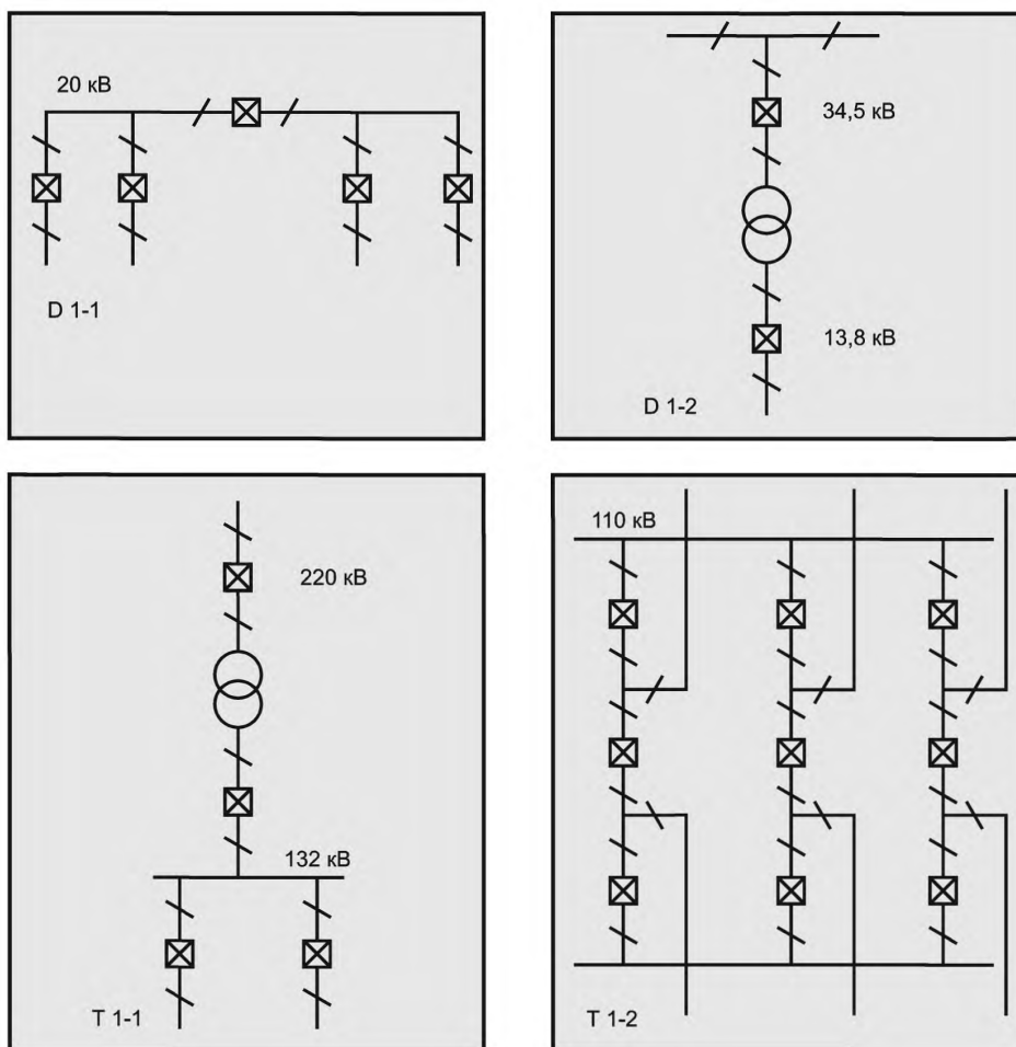
Рисунок 4 — Типы подстанций СН и ВН
