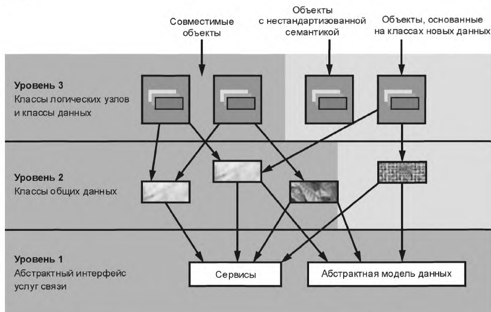
Рисунок 8 — Подход к моделированию в стандартах серии МЭК 61850
