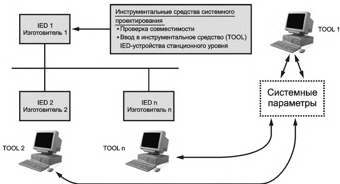
Рисунок 9 — Обмен системными параметрами
