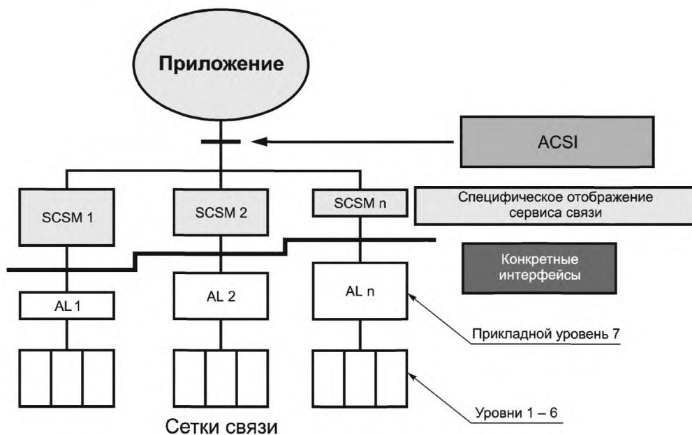
Рисунок 7 — Базовая эталонная модель
