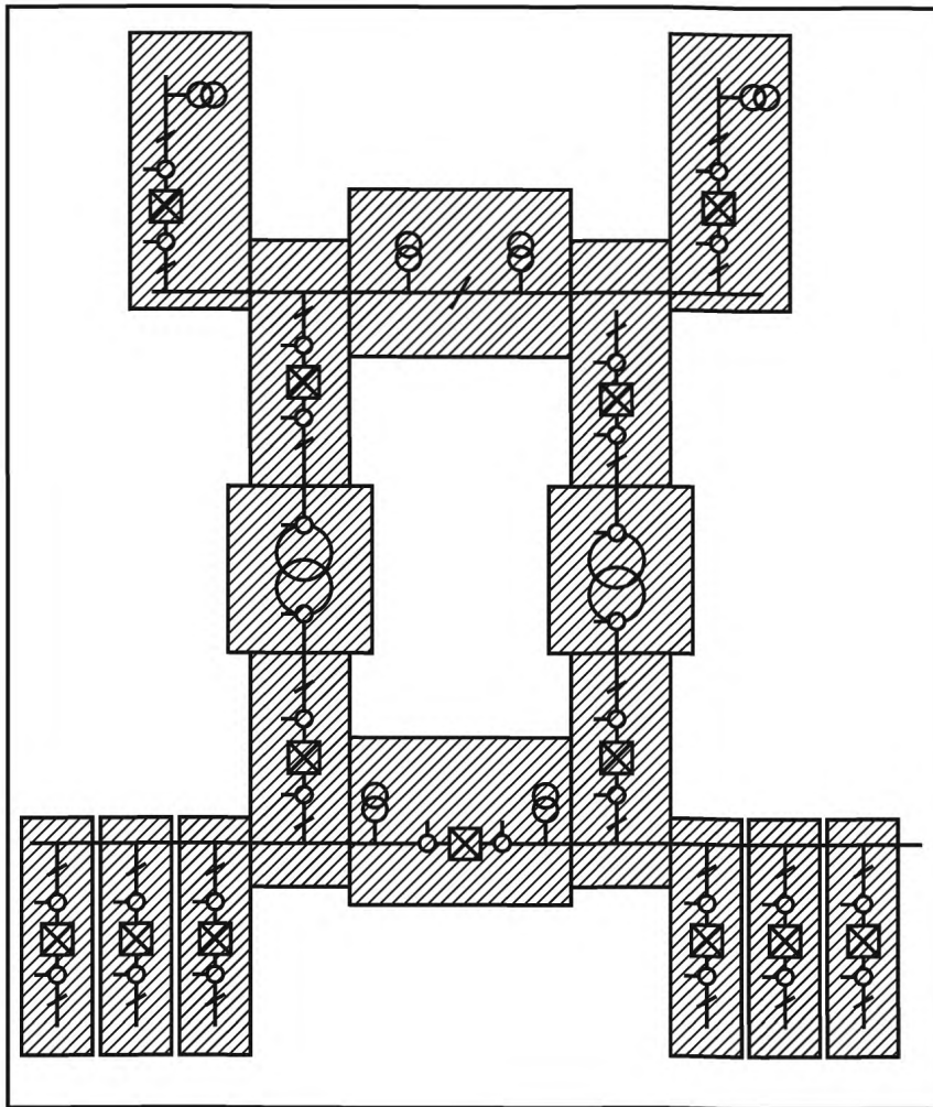
Рисунок А.7 — Деление на элементы присоединений (пример)
