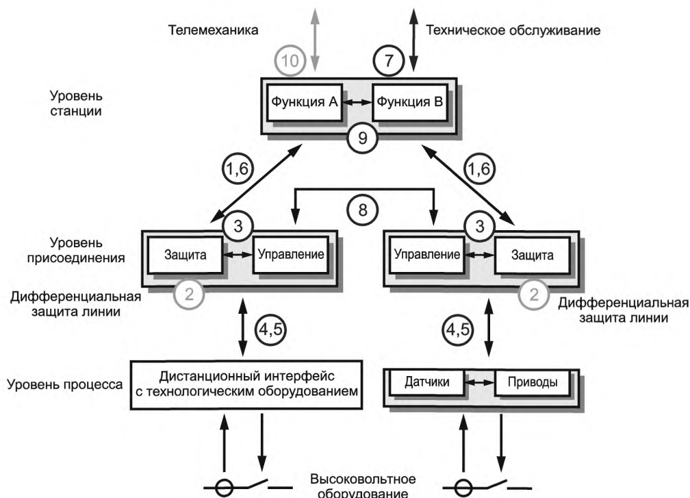
Рисунок 2 — Модель интерфейса системы автоматизации подстанции
