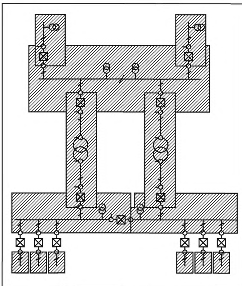
Рисунок А.8 — Типовые зоны защиты
