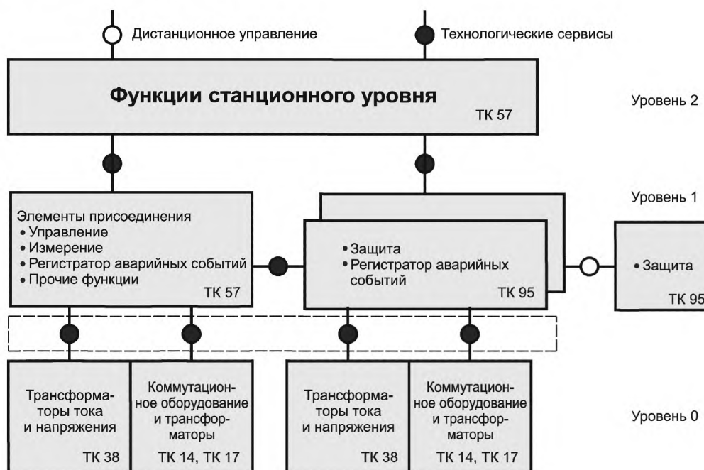
Рисунок 1 — Логические интерфейсы SA-системы
