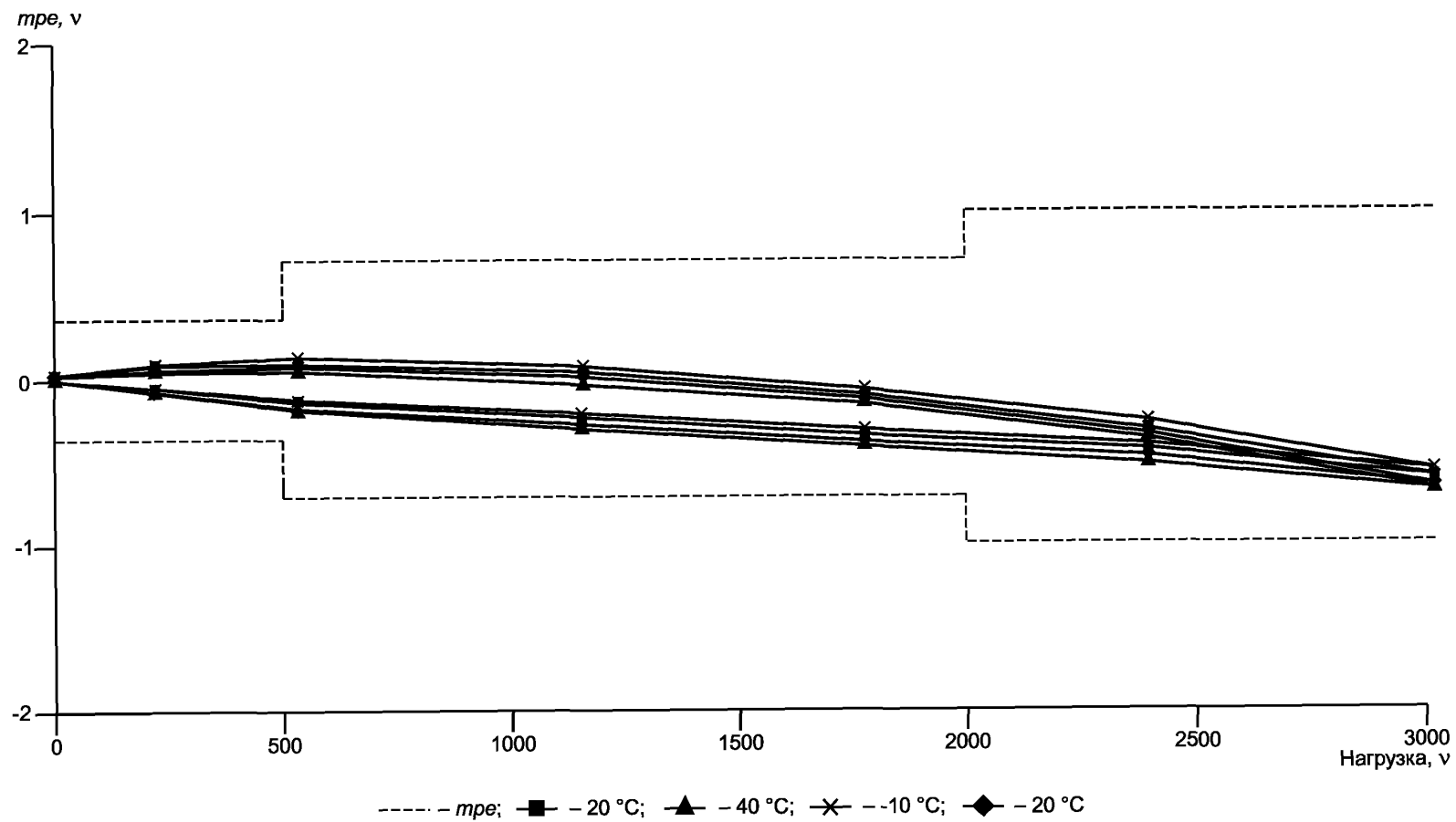
Рисунок Б.1 — Пример кривой погрешности
