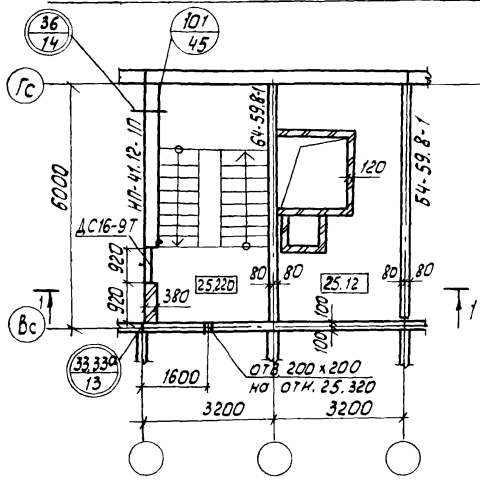
План машинного отделения на отм 25.220
