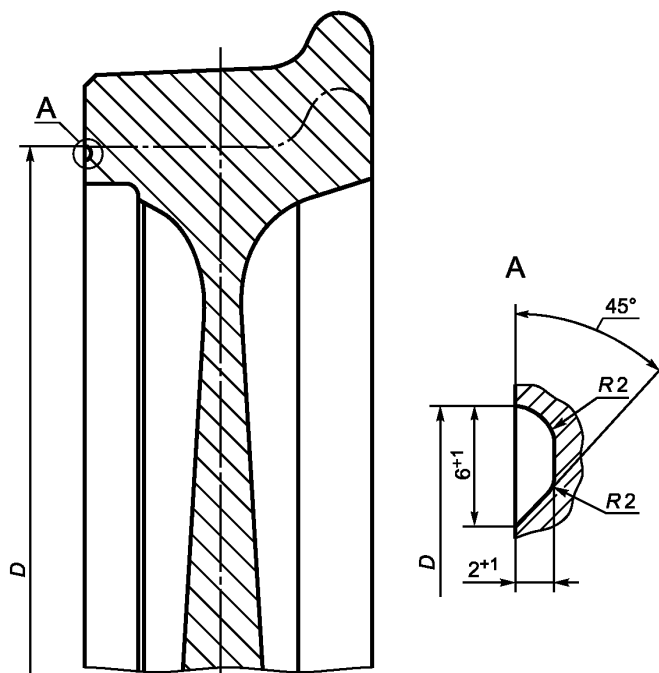
Рисунок 4 — Кольцевая проточка
