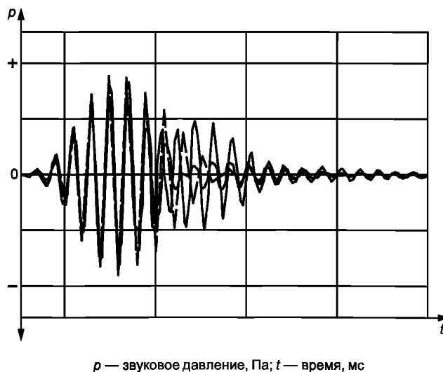
Рисунок 1 — Отражения узкополосного импульса, измеренные при трех разных ориентациях отражающей поверхности
